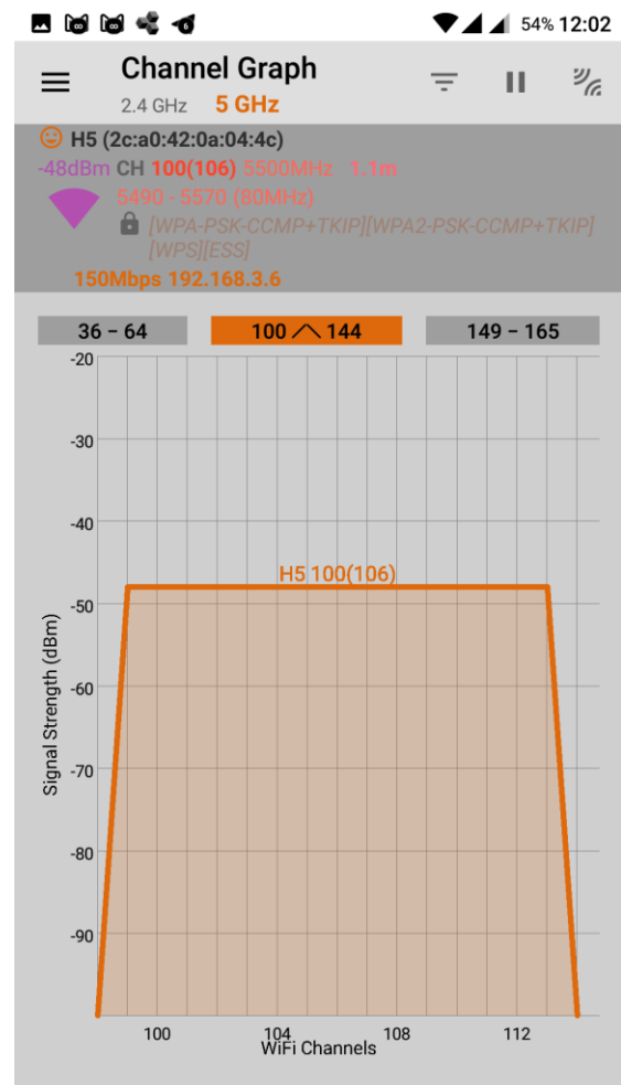
Рисунок 5.2 – Характеристики частотної смуги каналу 100 досліджуваної мережі
