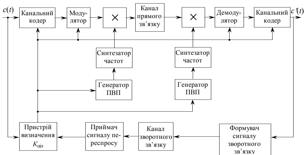
Рисунок 5 – Структурна схема системи передачі з ППРЧ зі структурною адаптацією
