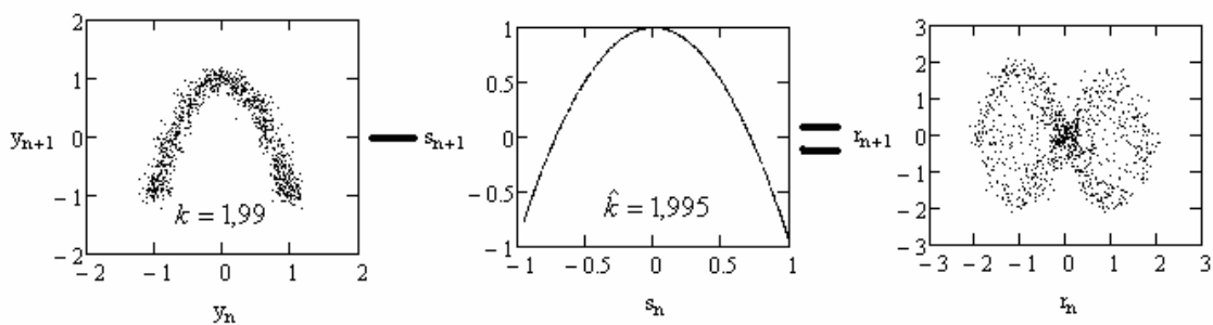
Рисунок 2 – Формирование фазового портрета разности наблюдаемой и ожидаемой последовательностей при \hat{k} \neq k_{uctm}
