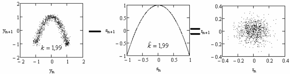
Рисунок 1 – Формирование фазового портрета разности наблюдаемой и ожидаемой последовательностей при \hat{k} = k_{uctm}
