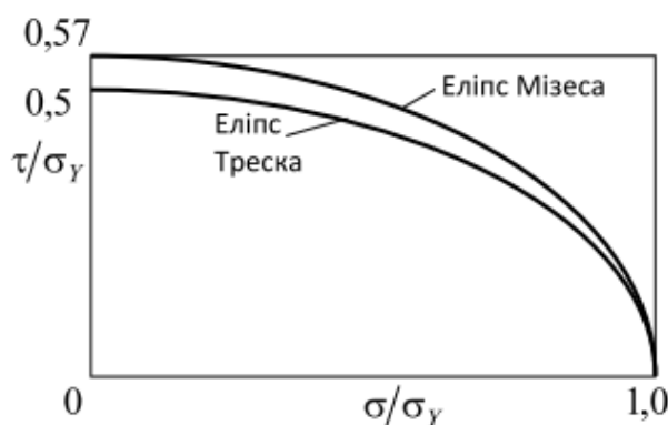
Рис. 8.2. Еліпси текучості Мізеса і Треска
