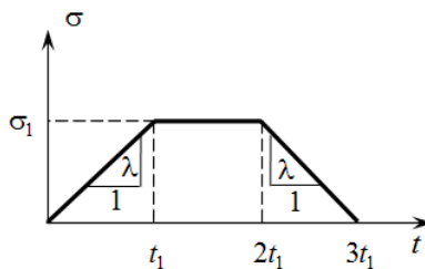
Рис. 9.12. Схема навантаження моделі Кельвіна
