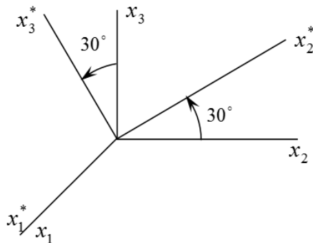
Рис. 3.8. Поворот навколо осі x_1 (до задачі 3.35)
