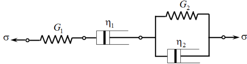
Рис. 9.4. Чотирьохпараметрична модель в'язкопружного середовища
