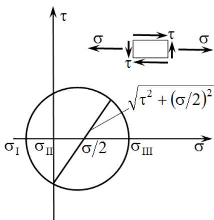
Рис. 8.1. Діаграма Мора
