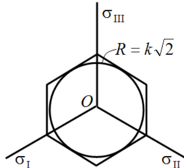
Рис. 8.16. Криві текучості, що відповідають критерию Треска
