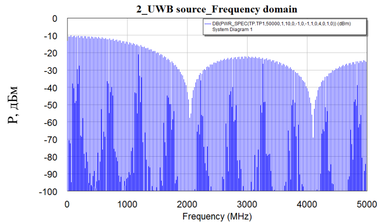
Рисунок 5 – Спектр надкороткого імпульсного сигналу на виході блоку PPULSE
