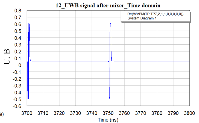
Рисунок 19 – Часова форма сигналу на виході змішувача передавального тракту (в масштабі 100 нс)
