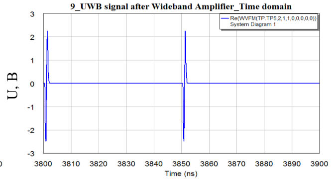
Рисунок 16 – Осцилограма гаусівського моноциклу на виході ланцюга «підсилювач-атенюатор» (в масштабі 100 нс)
