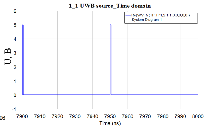
Рисунок 4 – Осцилограма надкороткого імпульсного сигналу на виході імпульсного генератору (в масштабі 100 нс)
