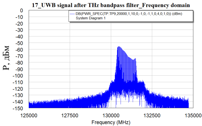
Рисунок 26 – Спектр IR-UWB сигналу на виході смугового фільтра передавального тракту радіолінії ТГц діапазону
