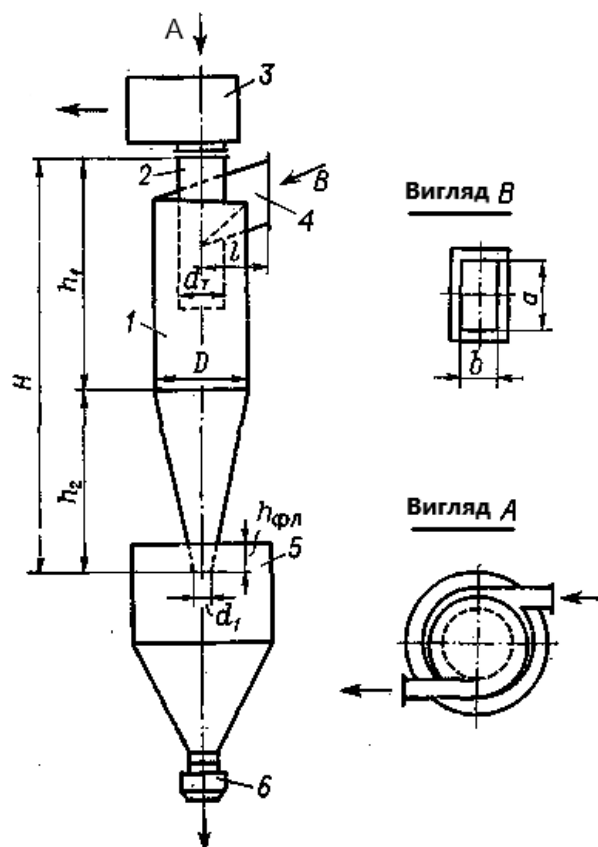
Рис. 5. Схема циклону: 1 - корпус; 2 - вихлопна труба; 3 - равлик; 4 - вхідний патрубок; 5 - приймальний бункер; 6 – засувка
