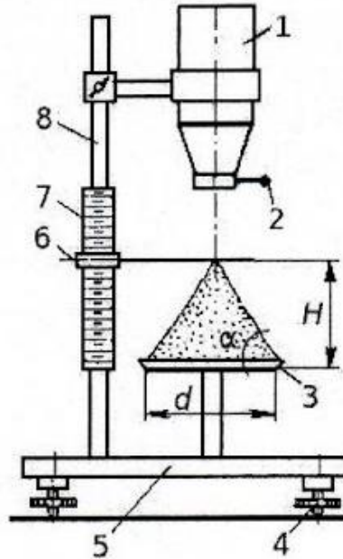
Рис. 3. Визначення кута природного відкосу методом насипання з воронки: \alpha - динамічний кут природного укосу, 1 - бункер, 2 - затвор, 3 - диск, 4 - регулюючі гвинти, 5 - підстава, 6 - пересувний покажчик, 7 - лінійка, 8 - штатив
