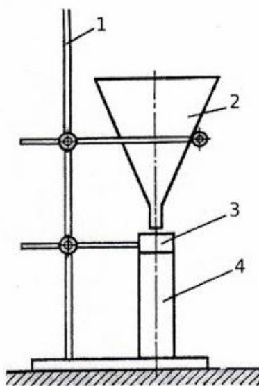
Рис. 2. Установка для вимірювання насипної щільності пилу: 1 - штатив, 2 - воронка, 3 - приймальне кільце, 4 - алюмінієвий циліндр
