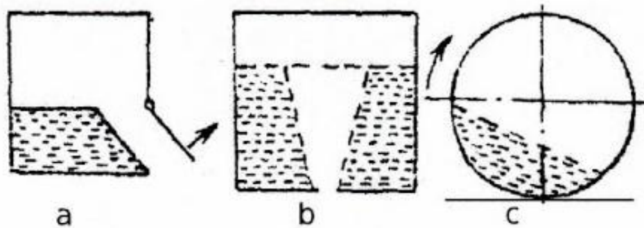
Рис. 4. Методи визначення кутів природного укосу і обвалення: а - висипанням з ємності при відкритті вікна, і - освітою кратера, з - обертанням ємності
