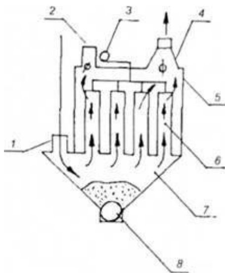
Рис. 8. Принципова схема рукавного протитічного пиловловлювача:
