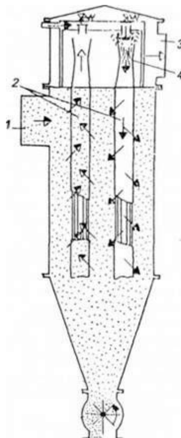
Рис. 9. Схема рукавного пиловловлювача з імпульсним продуванням:
