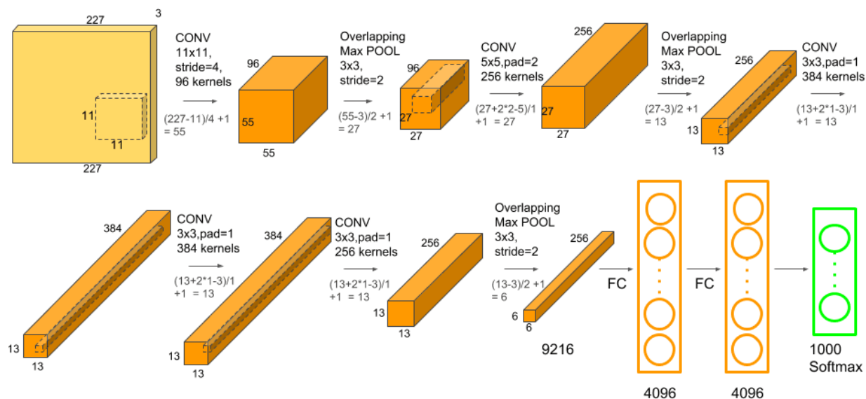
Рисунок 3.1. Структура AlexNet
