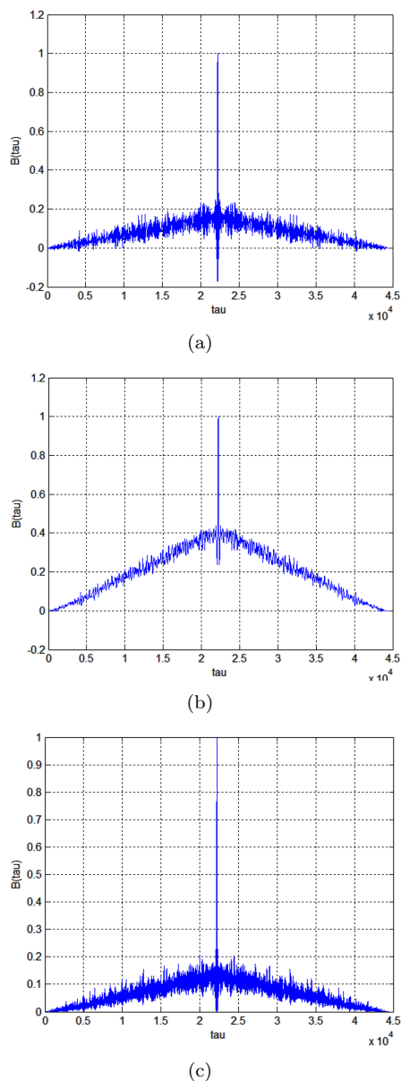
Рис. 3. Зображення цільової функції для розв'язків системи 1: (a) – розв'язок x ; (b) – розв'язок y ; (c) – розв'язок z .
