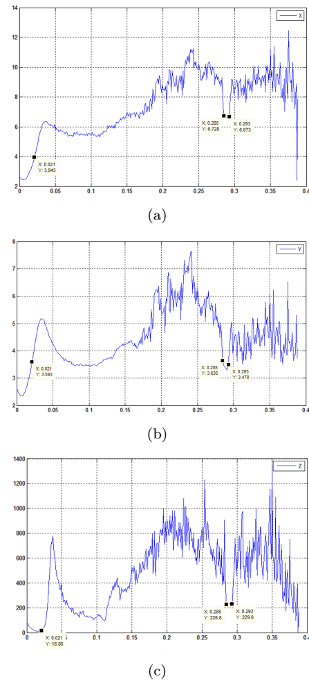
Рис. 2. Зображення цільової функції для розв'язків системи 1: (a) – розв'язок x ; (b) – розв'язок y ; (c) – розв'язок z .
