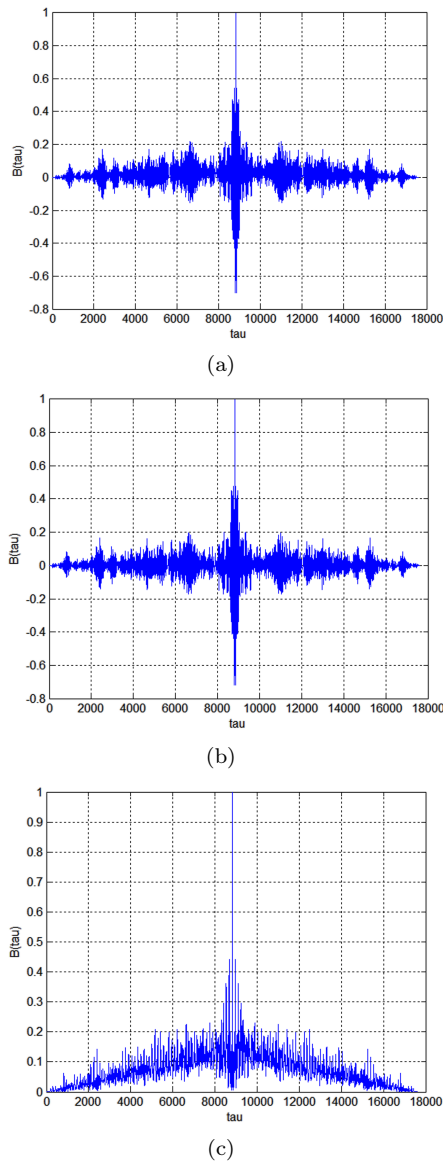
Рис. 1. Автокореляційна функція вихідних сигналів системи 1: (a) – сигнал x ; (b) – сигнал y ; (c) – сигнал z . функцію наступним чином [5]:
