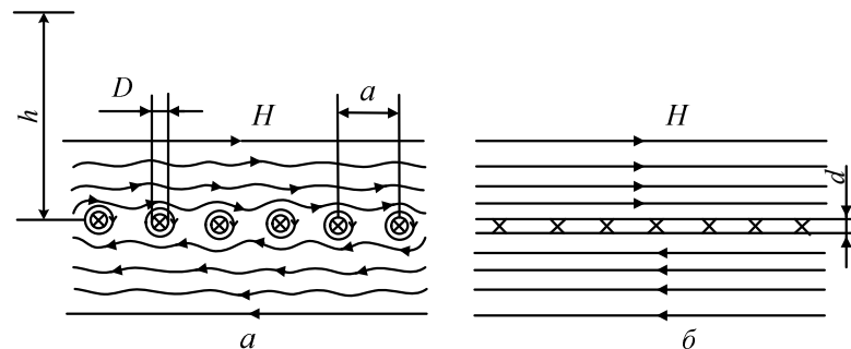
Рисунок 1 – Магнітне поле струмів, які протікають по сітці (а) та по суцільному екрану (б)
