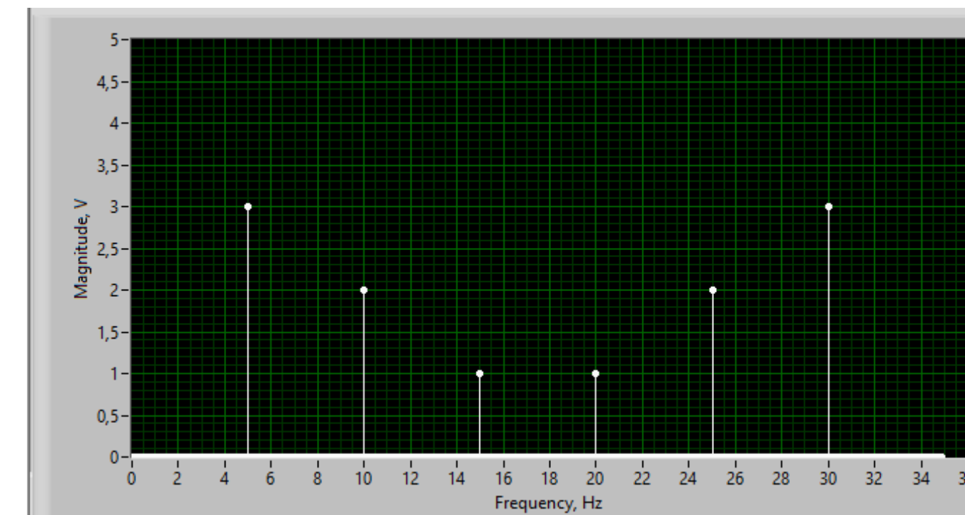
Спектр сигналу
