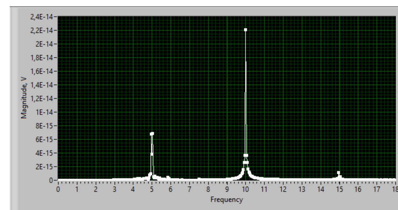
Різниця спектрів
