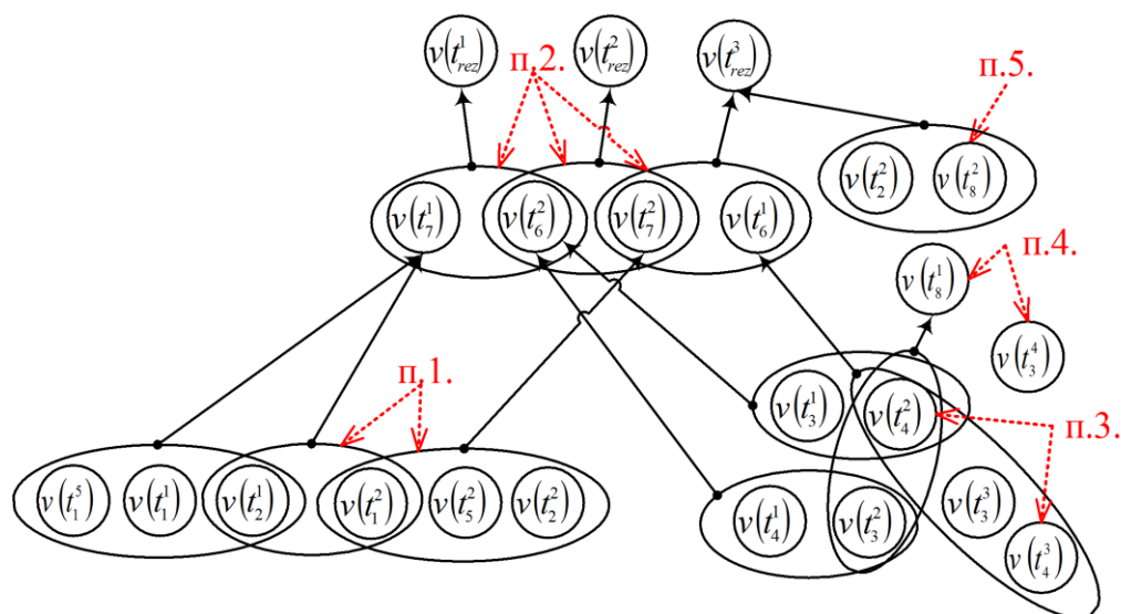
Рисунок 6. Пример метаграфа S^I , соответствующего БНЗ Мамдани, которая не является лингвистически полной
