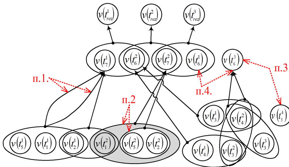
Рисунок 3. Пример метаграфа S' , соответствующего БНЗ Мамдани, в которой присутствует избыточность
