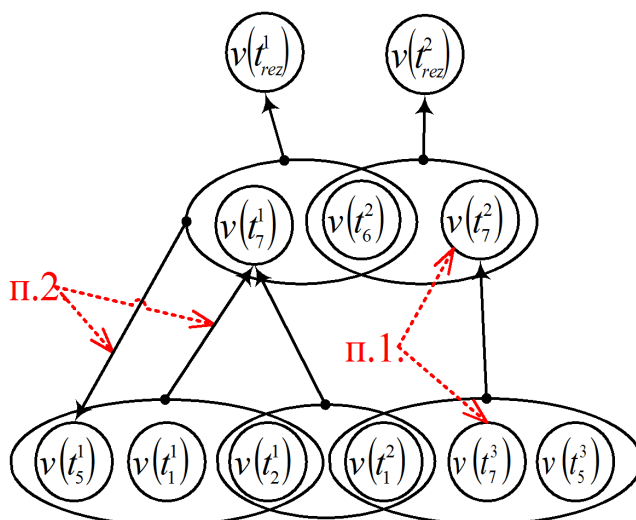
Рисунок 5. Пример метаграфа S^I , соответствующего БНЗ Мамдани, в которой присутствует заикливание
