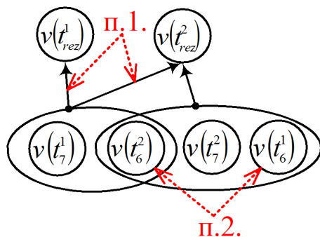
Рисунок 4. Пример метаграфа S' , соответствующего БНЗ Мамдани, которая является лингвистически противоречивой
