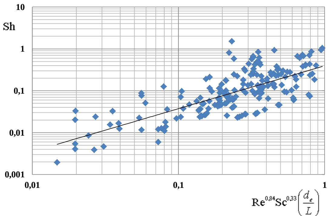
Рисунок 3.11 – Узагальнена критеріальна залежність
