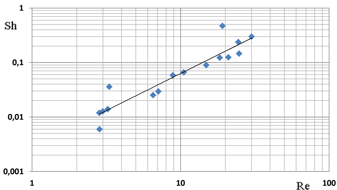
Рисунок 3.6 – Залежність критерію Шервуда від критерію Рейнольдса (діапазон зміни значень критерію Шмідта Sc = 1413 - 1615 )
