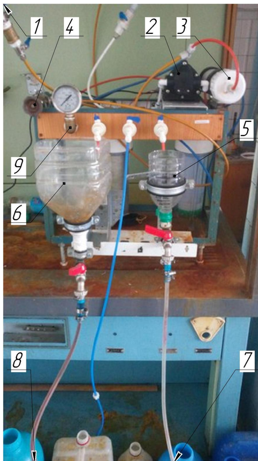
1 – ємність з початковим розчином; 2 – насос; 3 – мембранний апарат з рулонованим модулем; 4 – регулювальний кран; 5 – ємність вимірювання витрат пермеату; 6 – ємність для вимірювання витрат ретентату; 7 – збірник пермеату; 8 – збірник ретентату; 9 – манометр;
