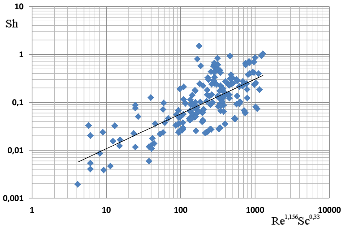
Рисунок 3.9 – Уточнення показника степеня при критерії Рейнольдса
