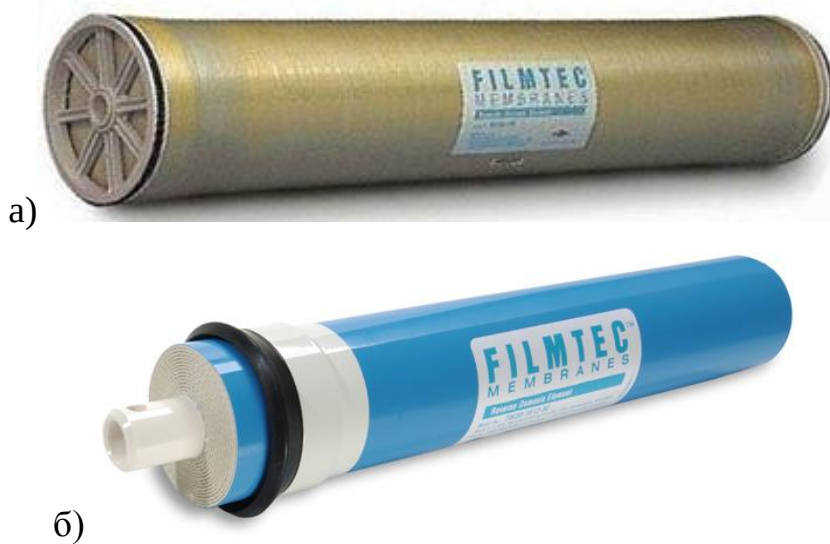
Рисунок 1.3 – Фотографії рулонованих мембранних модулів: (а) промислового, (б) побутового [44]
