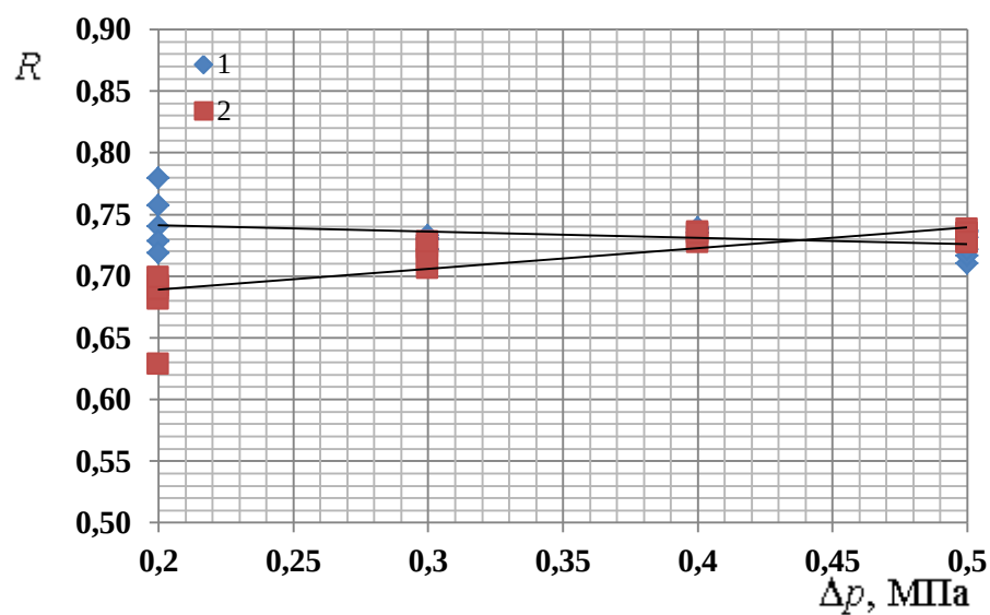
Рисунок 4.7 – Потік пермеату мембранного модуля Владіпор ОПМН – П
