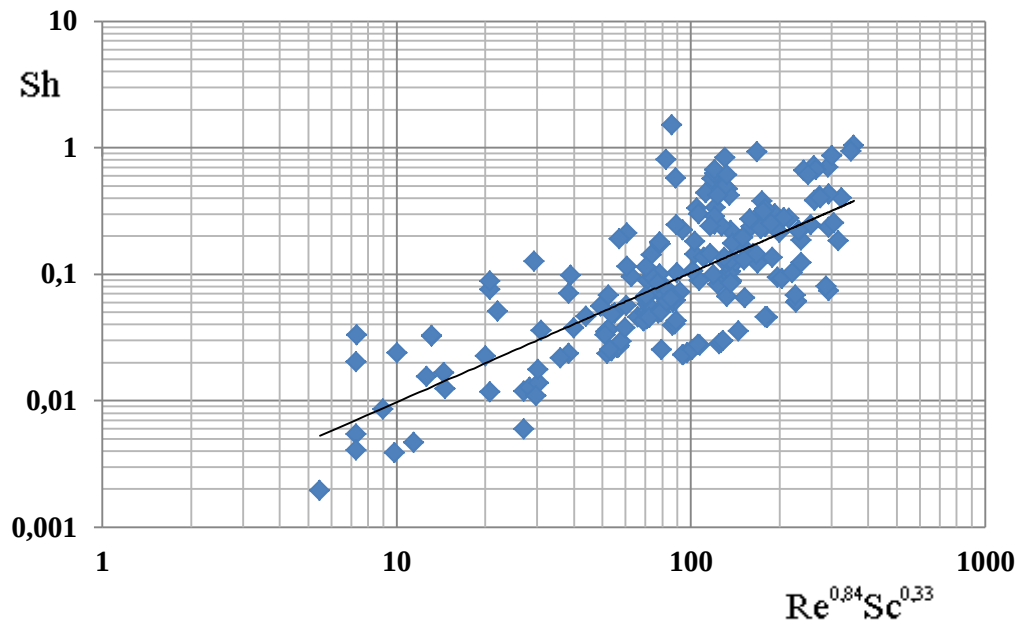
Рисунок 3.10 – Узагальнення результатів досліджень
