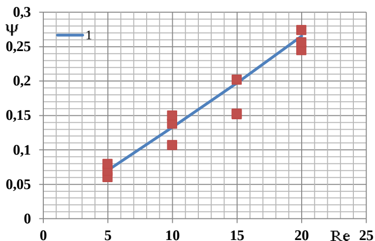
Рисунок 4.12 – Залежність коефіцієнта регенерації від критерію Рейнольдса
