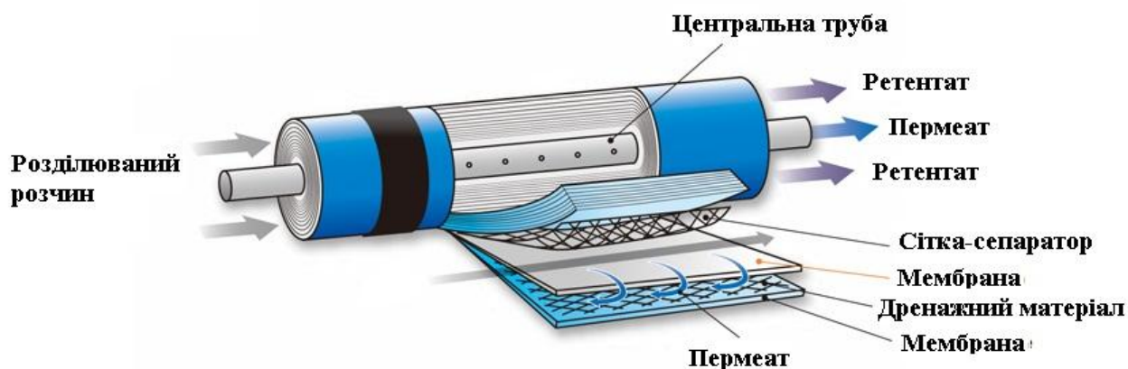
Рисунок 2.2 – Схема рулонового мембранного модуля [43]
