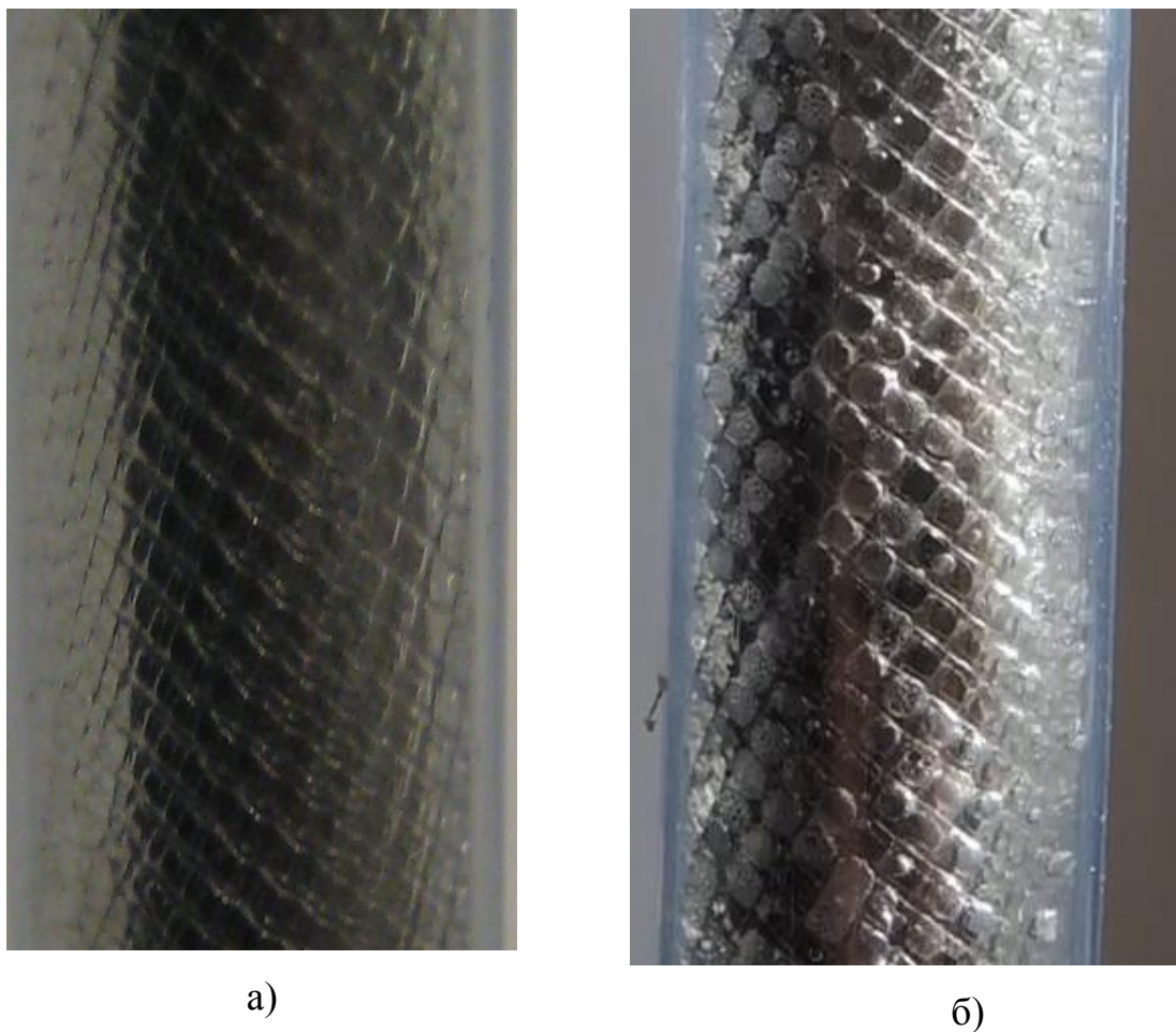
Рисунок 2.9 – Рух рідини в модельному каналі рулонованого мембранного модуля: а) при p = 0,06 МПа і t = 17 °С; б) при температурній кавітації p = 0,02\text{--}0,03 МПа і t = 45 °С.
