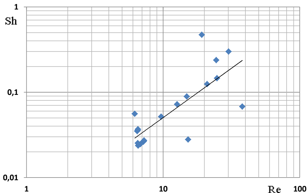
Рисунок 3.5– Залежність критерію Шервуда від критерію Рейнольдса (діапазон зміни значень критерію Шмідта Sc=1303 - 1491 )
