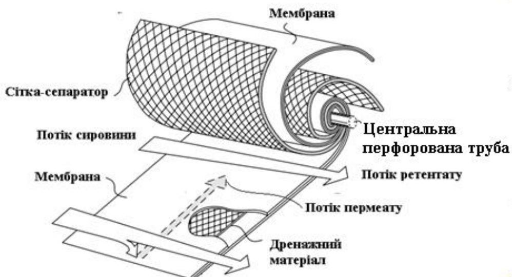
Рисунок 1.2 – Схема рулонового модуля [43]
