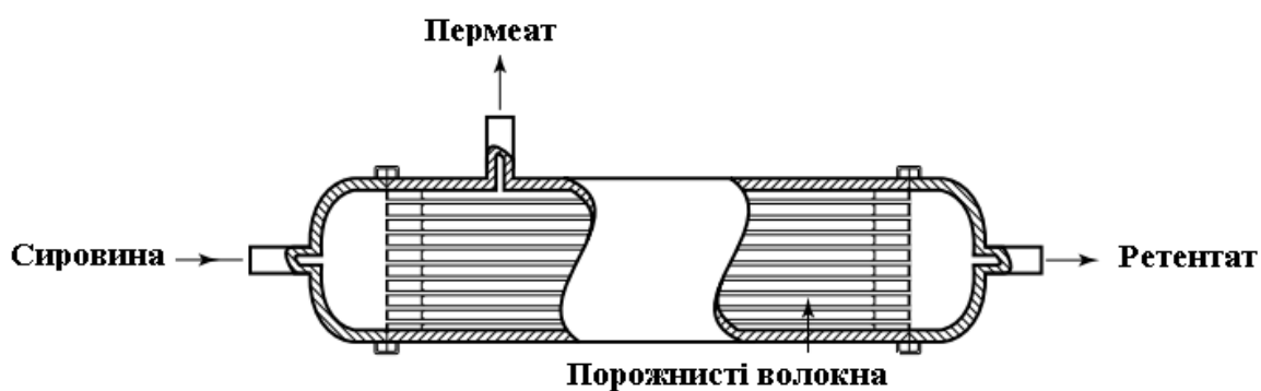
Рисунок 1.4 – Схема порожнистоволоконного мембранного модуля [43]
