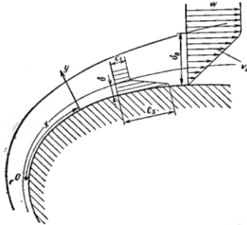
Рисунок 1.6 – Дифузійні та швидкісні шари на поверхні твердої частинки при масообміні з рідким середовищем [153]
