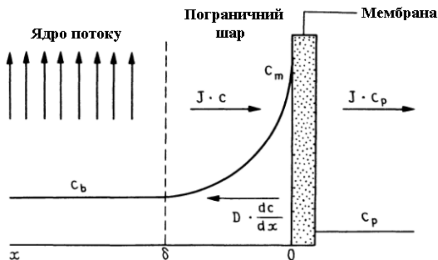
Рисунок 1.5 – Профіль концентрації в пограничному шарі мембрани за стаціонарного режиму концентраційної поляризації
