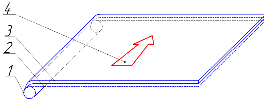
1 – центральна труба; 2 – сітка-сепаратор; 3 – пакет мембран; 4 – напрямок руху промивного розчину.
