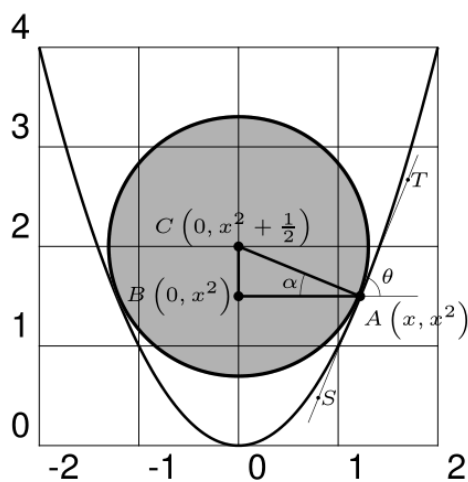
Рис. 1а. Взаємне розташування параболоїда та кулі, переріз площиною XOZ . Перший випадок.
