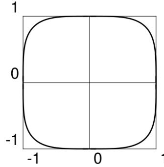
Рис. 3. Овал Ламе 4-го степеня
