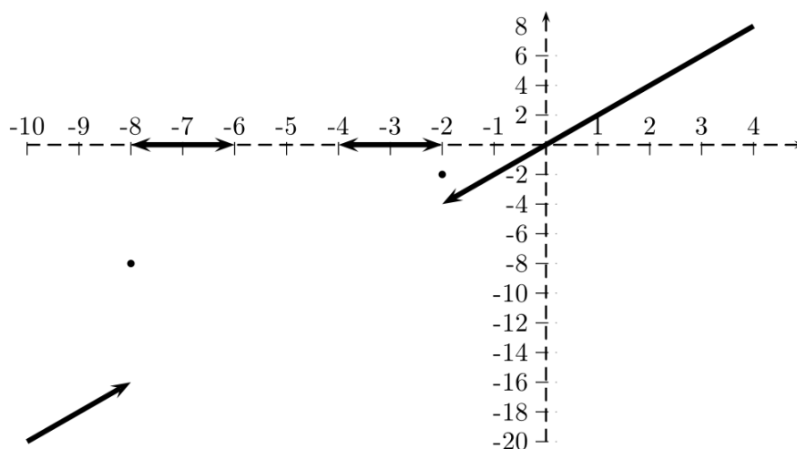
Рис. 2. Графік функції f(x)
