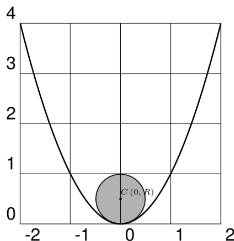
Рис. 1б. Взаємне розташування параболоїда та кулі, переріз площиною XOZ . Другий випадок.
