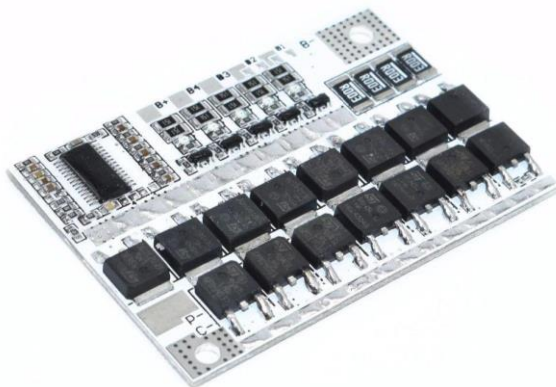
Рисунок 2.4 — BMS 4S 60-100A 12V Li-Pol [8]
