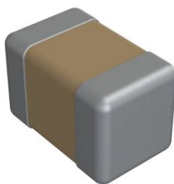
Рисунок 2.17 — 0805J0500221FCT
