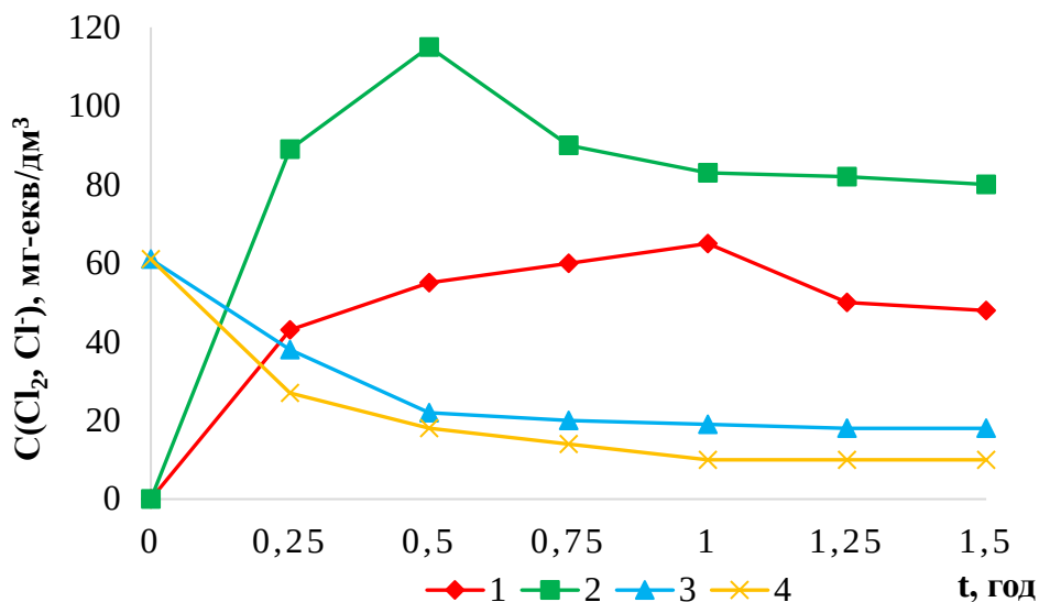
Рис. 2. Зміна концентрації сполук окисленого хлору (1 ; 2), хлоридів (3; 4) в анодній камері двокамерного електролізера ( мембрана-МА-41) з часом електролізу при концентрації хлоридів в анодній камері 61 мг-екв/дм 3 , лужності католіту 200 мг-екв/дм 3 , при анодній щільності струму, А/дм 2 : 4,17 (1; 3) та 8,33 (2; 4)
