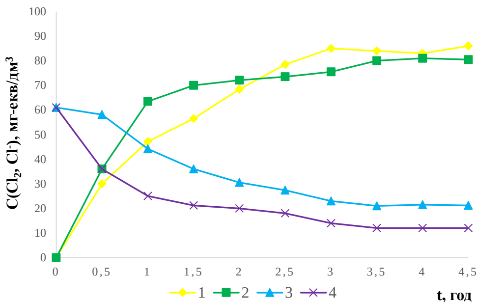
Рис. 1. Залежність концентрації сполук окисленого хлору (1; 2) та хлоридів (3; 4) від часу електродолізу при щільності струму А/дм 2 : 0,83 (1; 3) та 1,67 (2; 4) в анодній камері двокамерного електродолізера (мембрана МА-41) при концентрації хлоридів в анодній камері 61 мг-екв/дм 3 та лужності в катодній камері 200 мг-екв/дм 3
