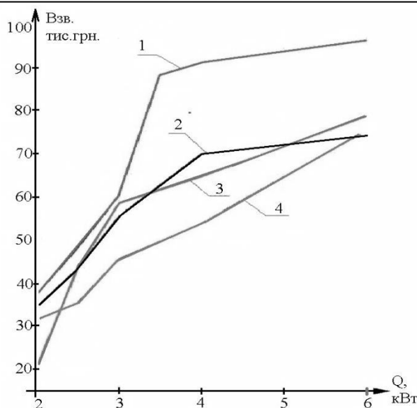
Рис.2. Залежність зведених витрат ( B_{зв} ) від холодопродуктивності спліт-систем ( Q ): 1 – 4 номери постачальників
