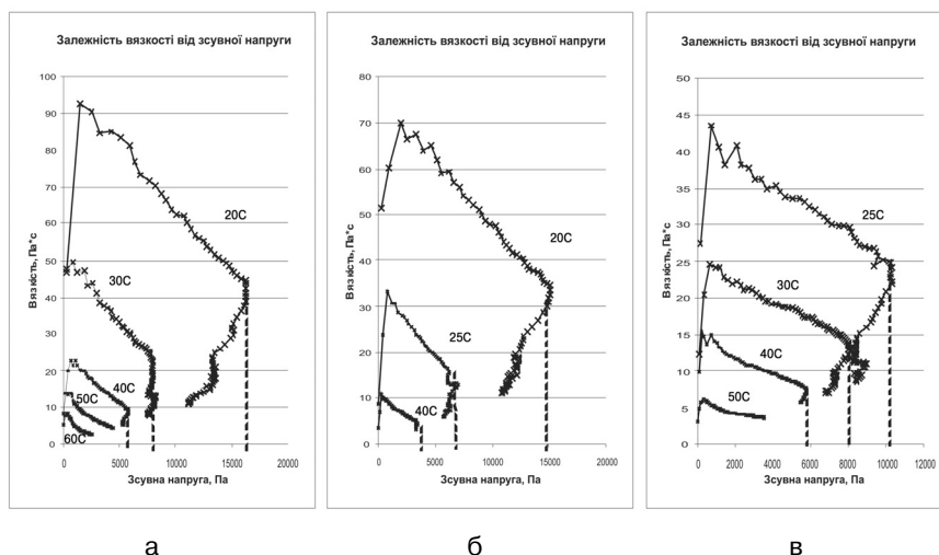
Рис. 4. Залежність в'язкості червоної фарби від зсувної напруги при різних температурах (вказані біля кожної з кривих): а — тиксотропних (негомogenізованих); б — гомогенізованих (ретельно перемішаних) фарб; в — взірці з середини верхньої половини тароупаковки (неперемішані)
