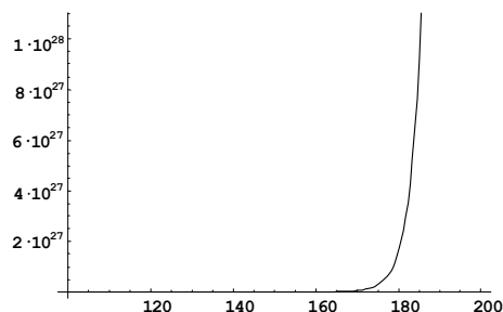
Рисунок 2 – Сложность атаки для преобразований в группе точек на эллиптической кривой
