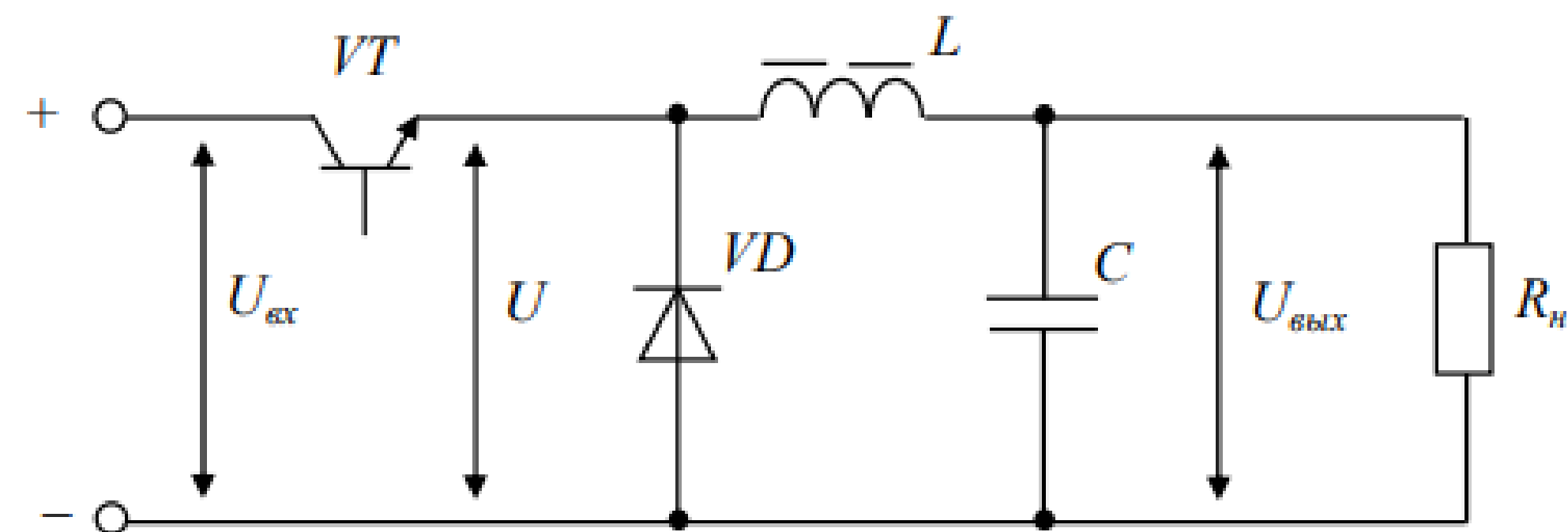
Класичний перетворювач
