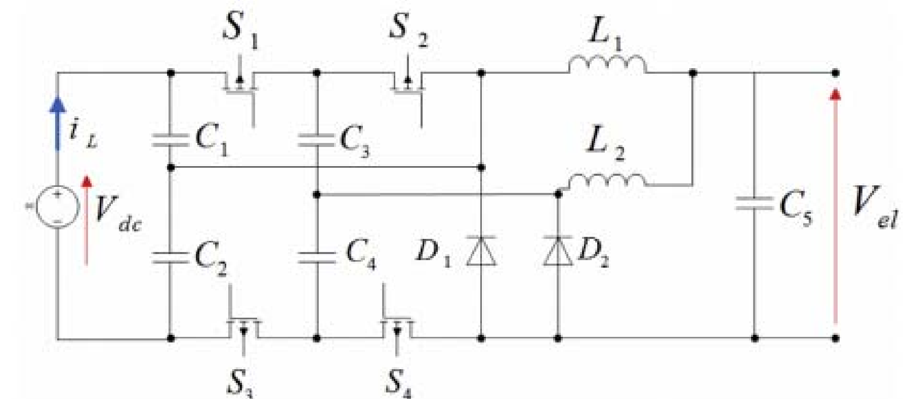
Схема з розширеним робочим циклом
