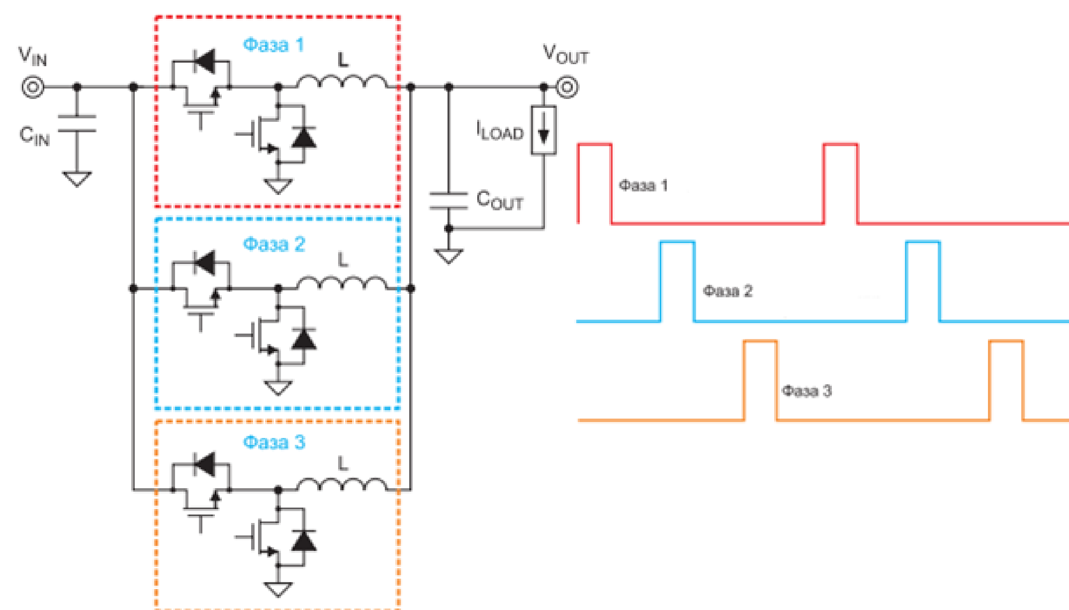
Багатофазний перетворювач
