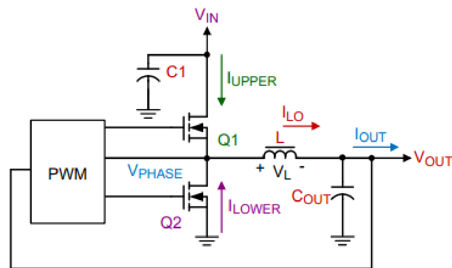
Синхронний перетворювач
