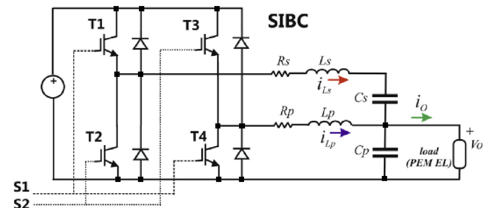
Схема перетворювача з компенсуючою фазою
