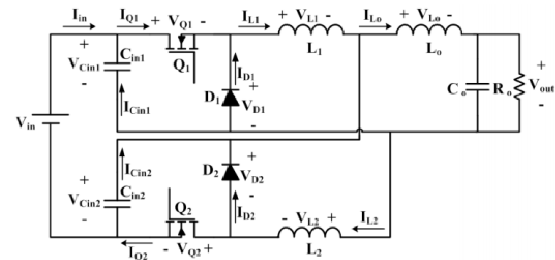
Перетворювач з надзвичайно низькими пульсаціями вихідного струму
