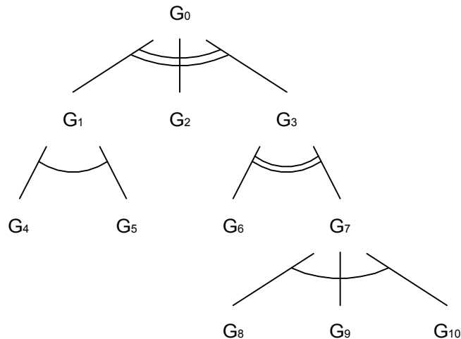
Рисунок 4 – Пример дерева атаки на цель G_0
