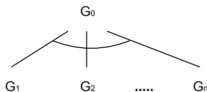
Рисунок 2 – И-декомпозиция
