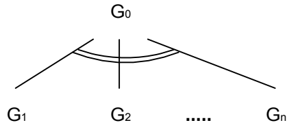
Рисунок 3 – ИЛИ-декомпозиция
