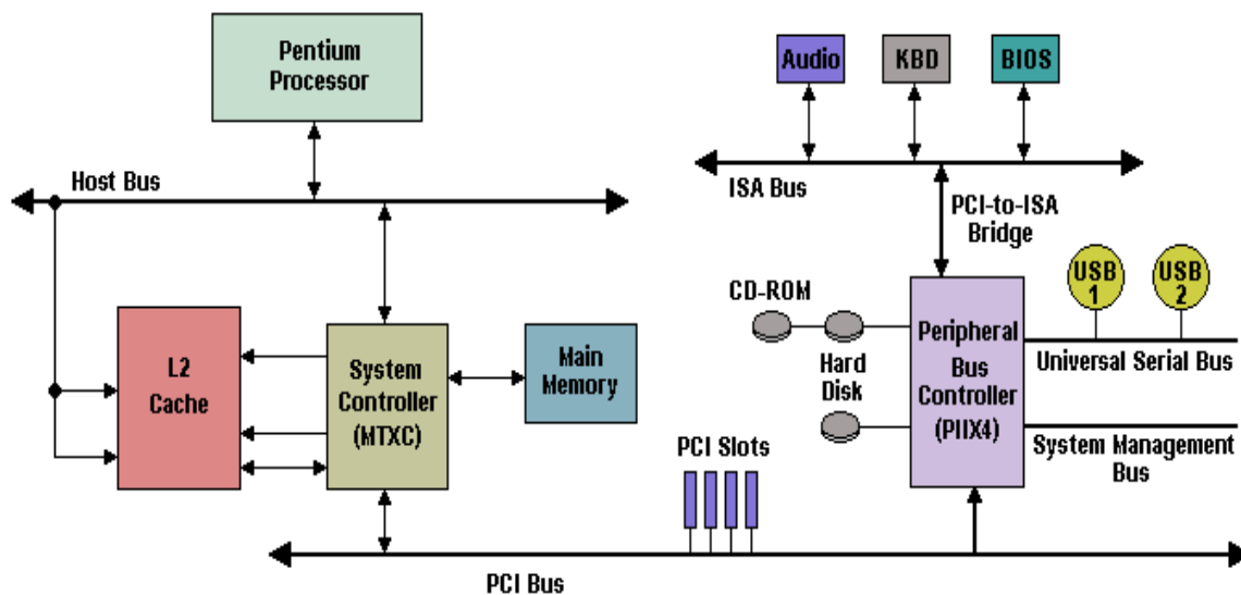
Рисунок 1 – Обобщённая структура компьютера на базе процессоров Pentium
