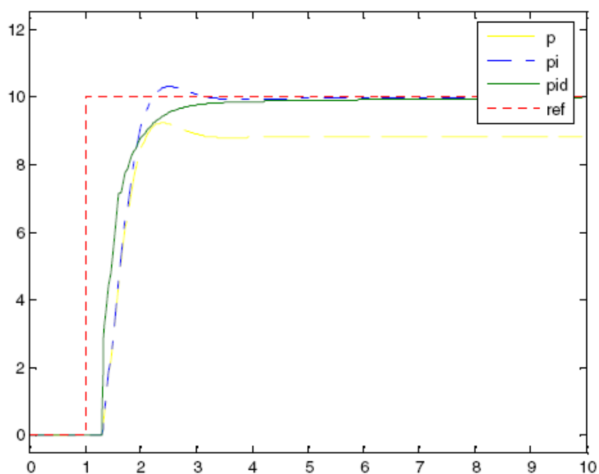
Рисунок 1.24 – Відгук П-, ПІ- та ПД-регулятора на сходинкову зміну опорного сигналу
