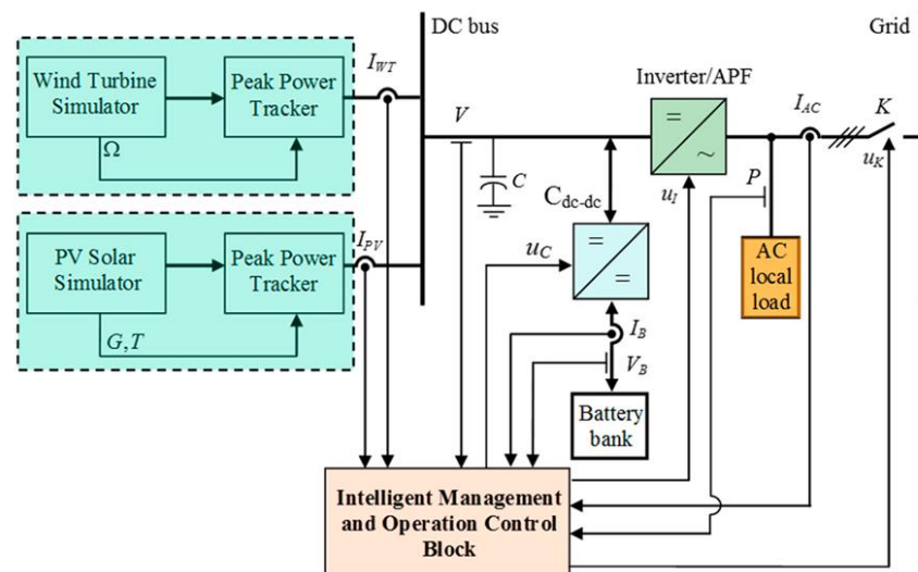
Рисунок 1.17 – Спрощена блок-схема, що ілюструє структуру енергорозподіленої системи [17]
