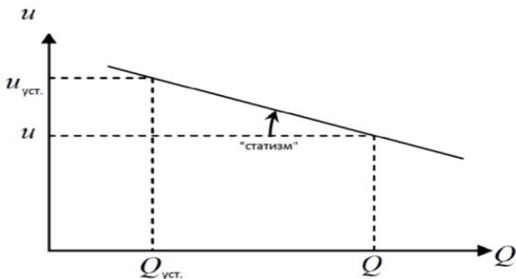
Рисунок 1.3- Регулювання напруги за допомогою коефіцієнта статизму [2]
