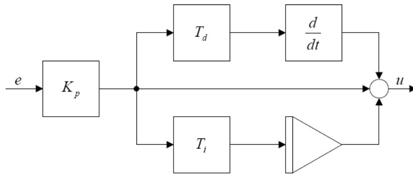
Рисунок 1.20 – Схема ПД-регулятора
