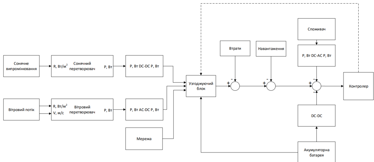
Рисунок 2.2 – Функціональна схема системи керування розподілом джерел енергозабезпечення підприємства
