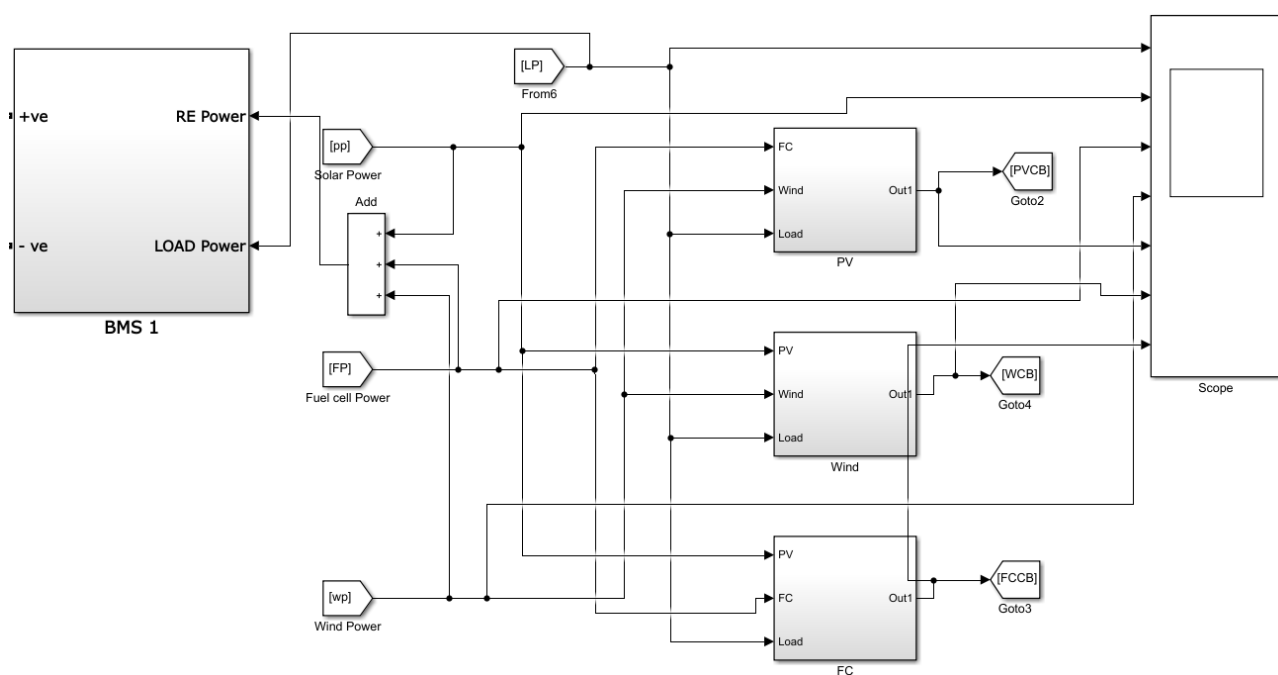
Рисунок 3.11 – Схема силового комутатора
