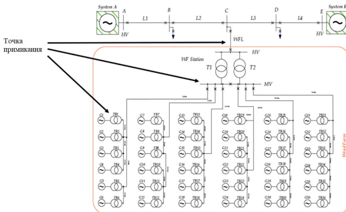
Рисунок 1.6 - Приклад моделі ВЕС в складі ЕС [2]
