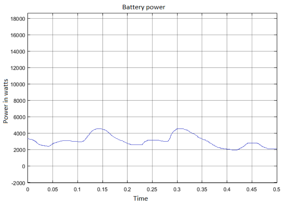
Рисунок 3.16 – Результати моделювання для АКБ (зима)
