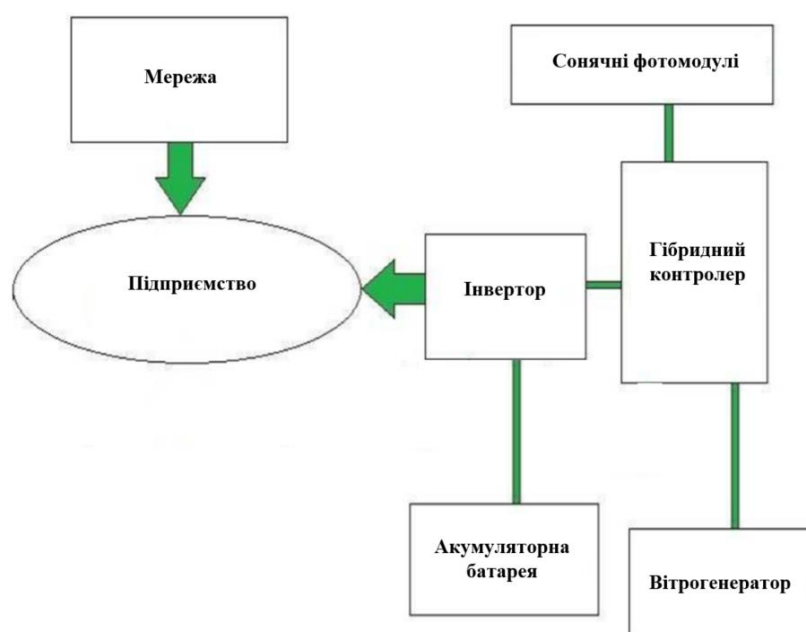
Рисунок 1.11 – Приклад системи енергозабезпечення з застосуванням ВДЕ
