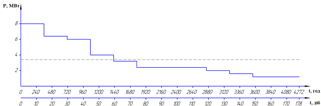
Рисунок 3.12 – Зимовий графік навантаження заводу
