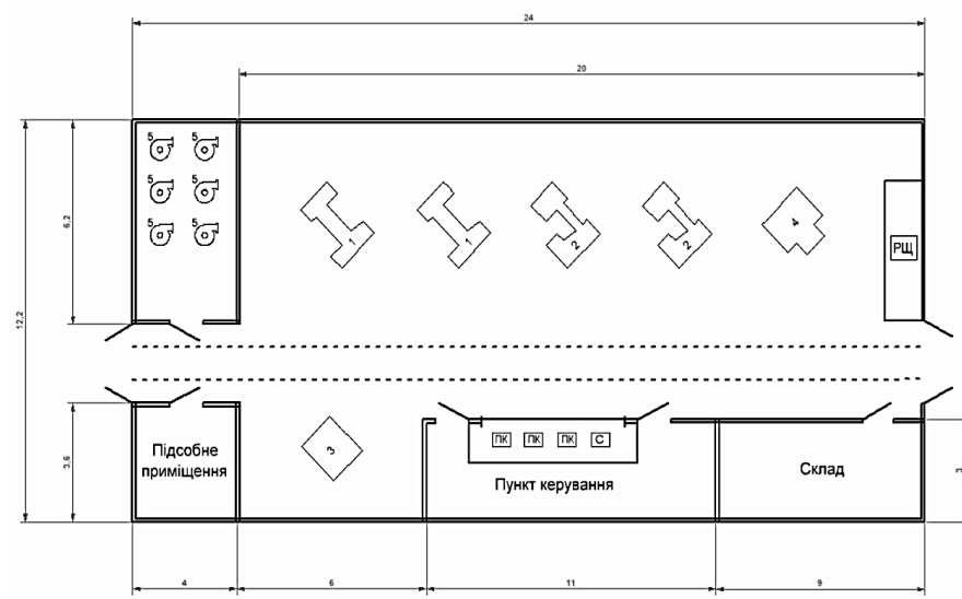
Рисунок 1.27 – План розташування обладнання заводу
