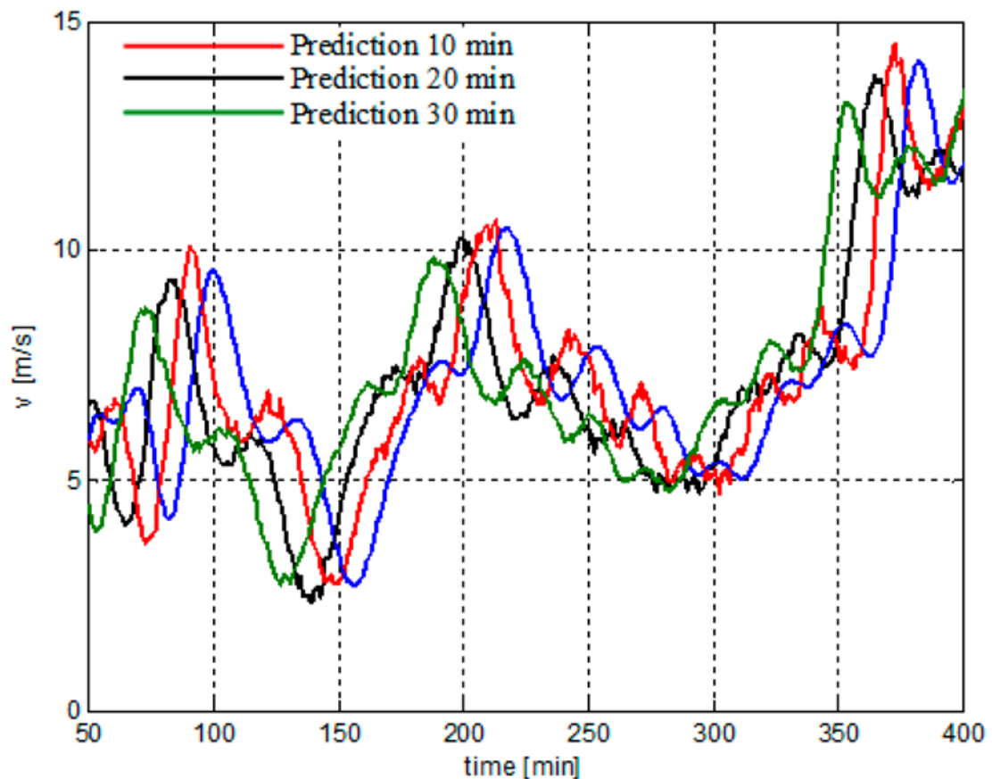
Рисунок 1.25 – Прогнозування швидкості вітру у системі керування [17]
