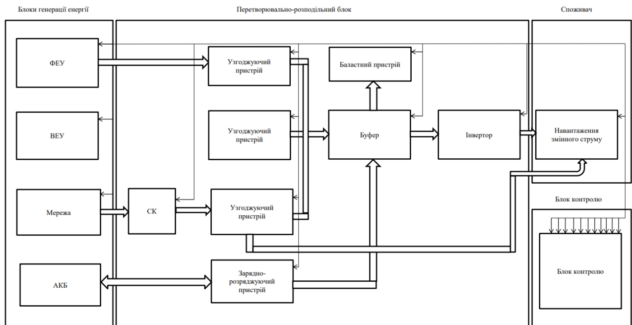
Рисунок 2.1 – Структурна схема системи керування розподілом джерел енергозабезпечення
