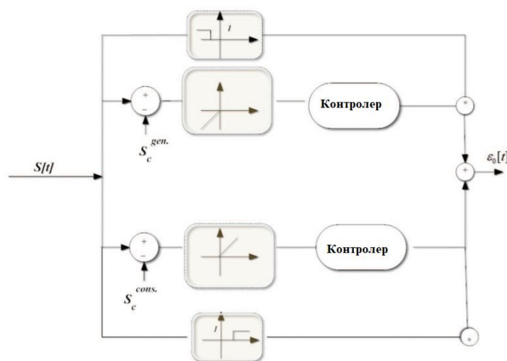
Рисунок 1.18 - Функціональна схема системи керування розподілом джерел енергозабезпечення
