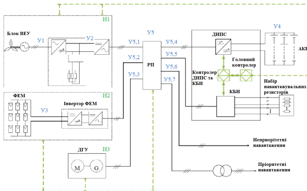
Рисунок 1.16 – Приклад функціональної схеми системи керування [7]
