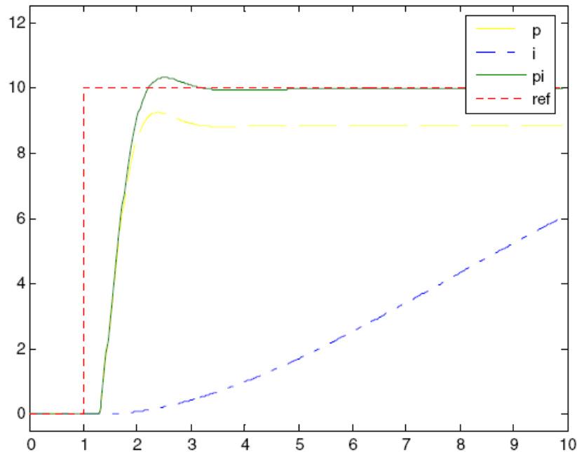
Рисунок 1.22 – Відгук І- та ІІ-контролера на сходишкову зміну опорного сигналу
