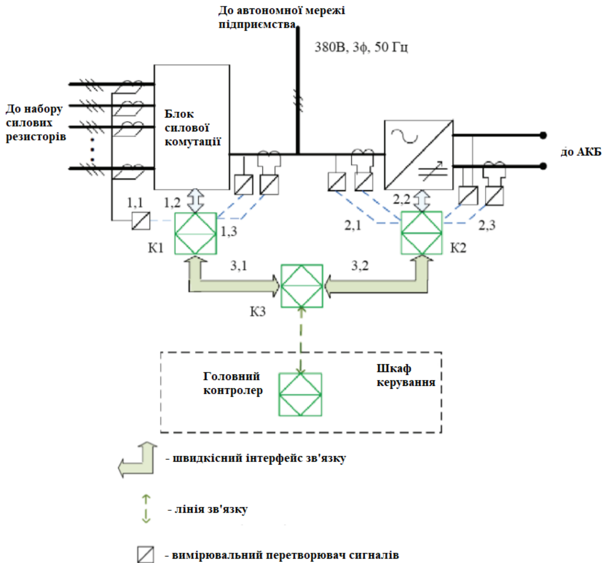
Рисунок 1.12 – Приклад функціональної схеми системи керування розподілом джерел енергозабезпечення підприємства [7]
