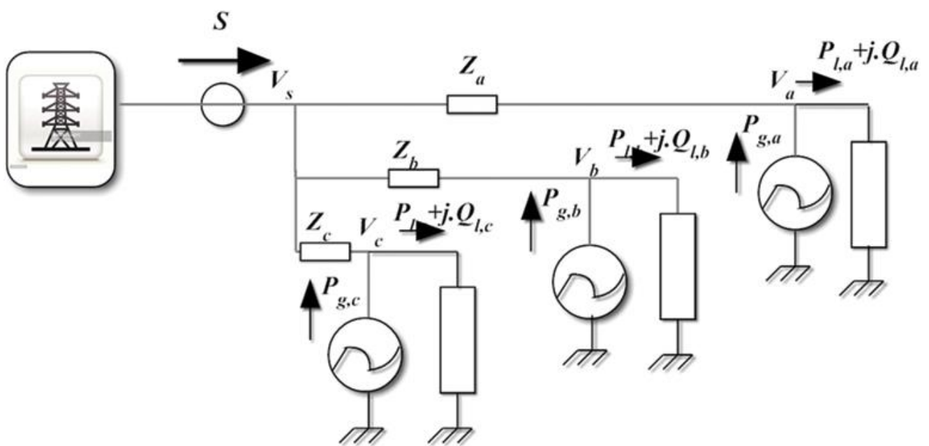
Рисунок 1.13 – Однолінійна схема розподільчої мережі [8]
