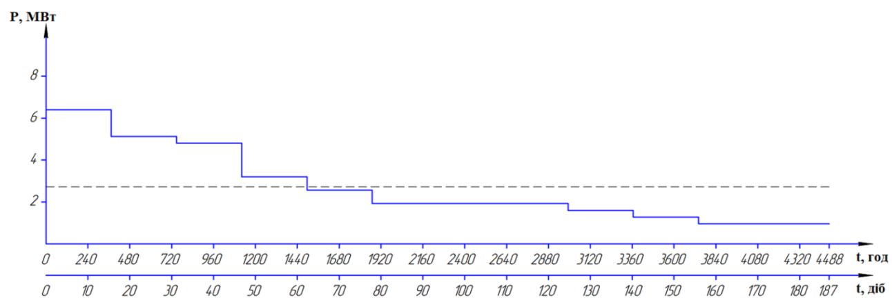
Рисунок 3.13 – Літній графік навантаження заводу
