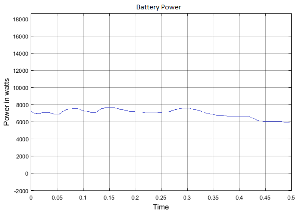
Рисунок 3.18 – Результати моделювання для АКБ (літо)
