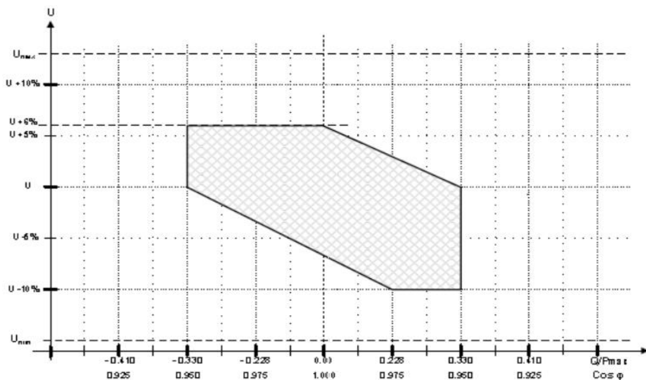
Рисунок 1.5 - Приклад регулювання напруги [2]
