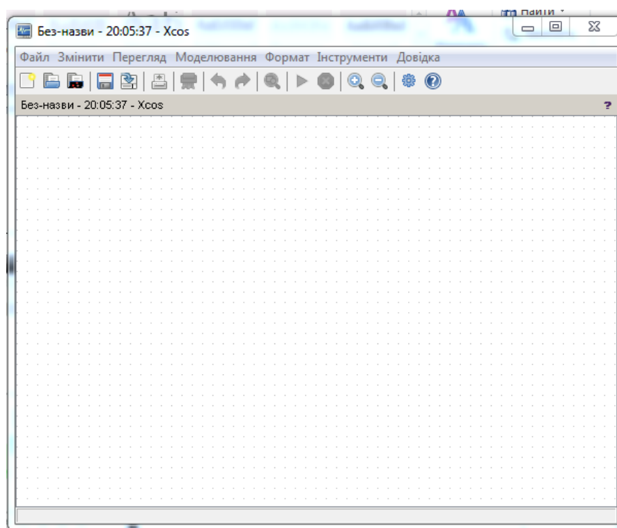
Рисунок 3.3 – Вікно редактора
