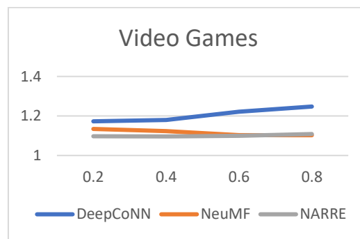
Рисунок 18 – Залежність MSE від Dropout для датасету Video Games
