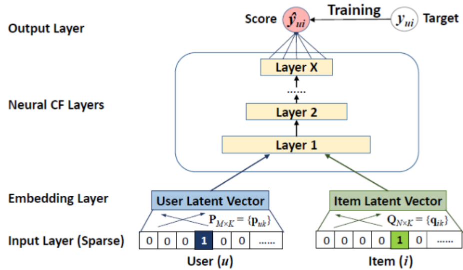
Рисунок 1 – Архітектура моделі Neu-CF
