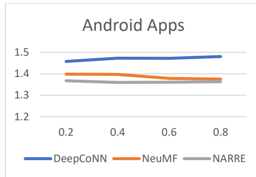
Рисунок 17 – Залежність MSE від Dropout для датасету Android Apps
