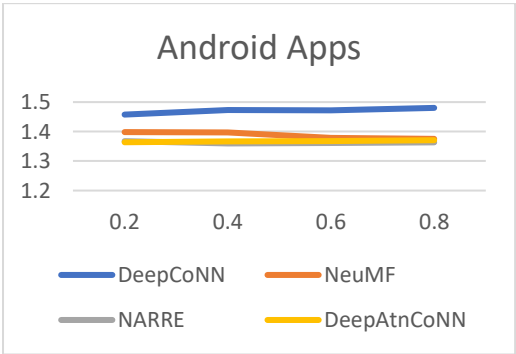
Рисунок 57 – Залежність MSE від Dropout для датасету Android Apps
