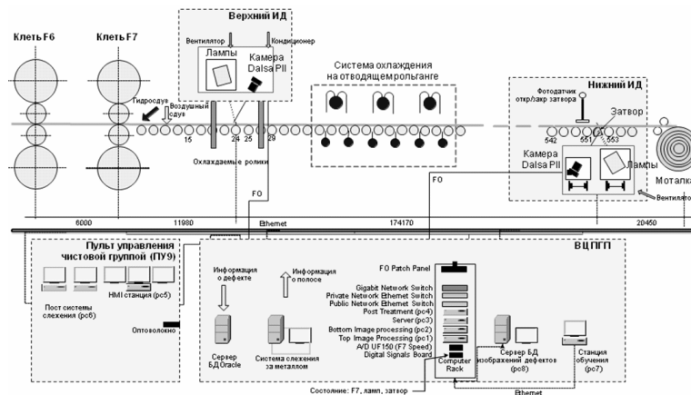
Рис. 1. Размещение оборудования СККП
