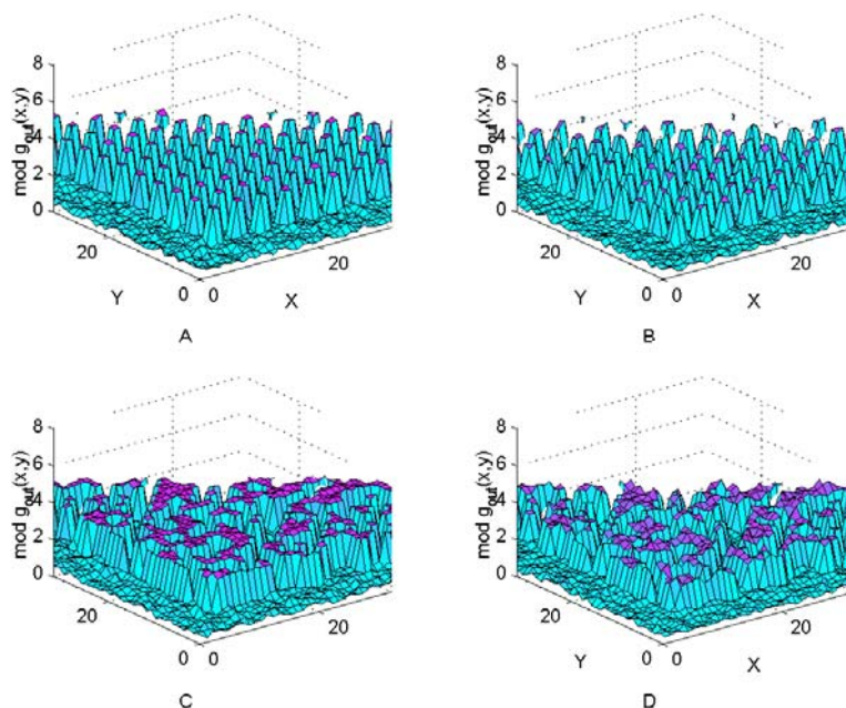
Рисунок 3 – Восстановленные изображения объектов, приведенных на рисунке 2 А, В, при синтезе киноформа А, С – предложенным методом; В, D – “error-reduction” методом.
