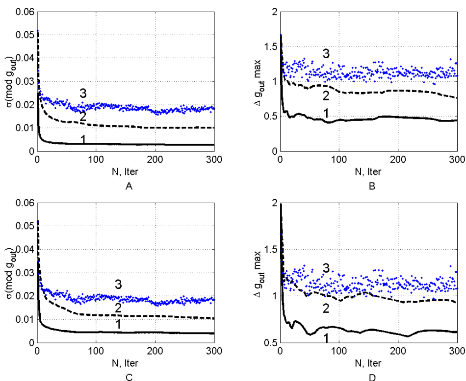
Рисунок 4 – Зависимость дисперсии и размаха амплитуды восстановленного изображения от номера итерации. А, В – для объекта изображенного на рисунке 2 А; С, D – для объекта изображенного на рисунке 2 В; 1 - предложенный метод; 2 – “error-reduction” метод; 3 – “input-output” метод [5]
