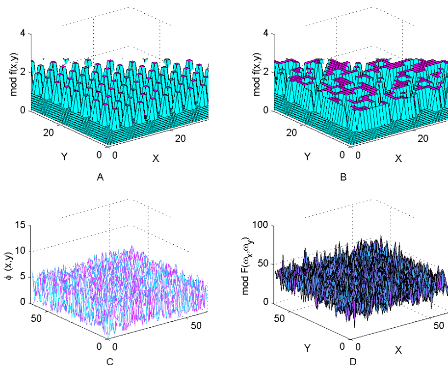
Рисунок 2 – Объекты: А – регулярная бинарная структура; В – случайная бинарная структура; С – объектно-ориентированный фазовый рассеиватель; D – оптимизированное амплитудное распределение в плоскости киноформа
