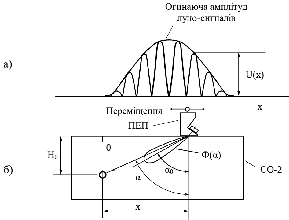
Рис. 3.1. Огибающая амплитуд луно-сигналов
