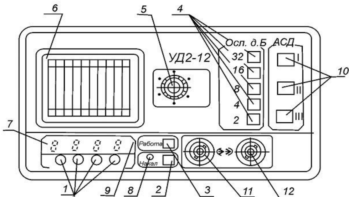
Рис. Д.2. Передня панель дефектоскопа УД2-12
