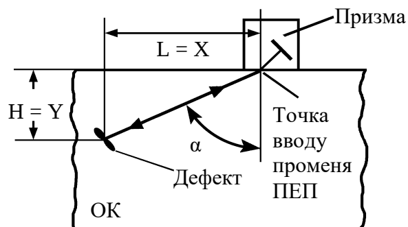
Рис 4.2. Схема приймання відбитого сигналу для похилого ПЕП
