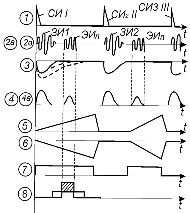
Рис. Д.5. Діаграми напруг
