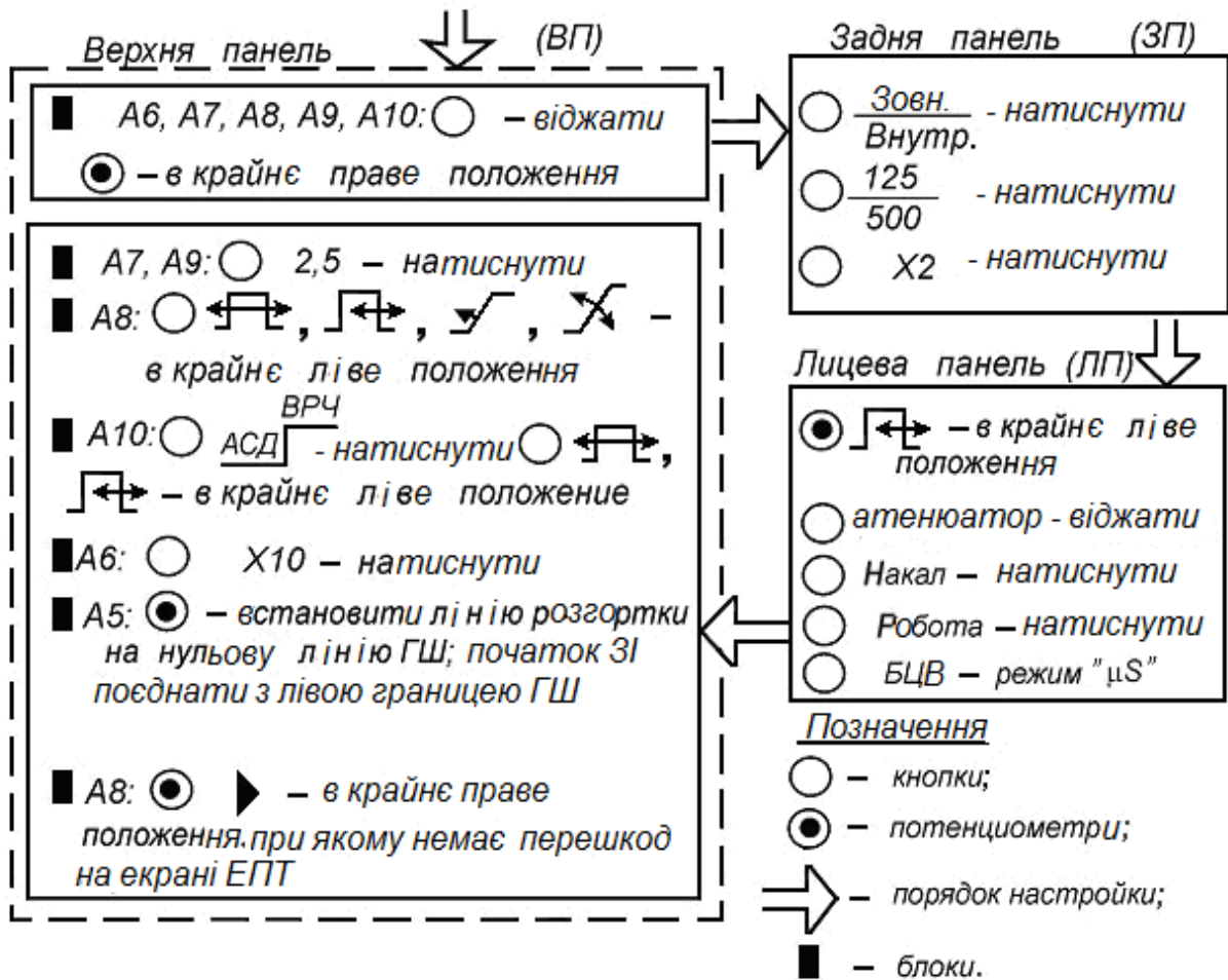
Рис. Д.3. Технологічна карта настроювання дефектоскопа
