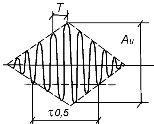
Рис. Д.6. Форма зондувальних імпульсів
