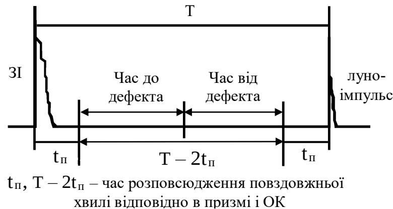
Рис. 4.3. Імпульси на екрані дефектоскопа для похилого ПЕП
