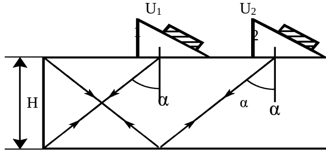
Рис. 2.1. Схема прозвучування зразка висотою H поперечною хвилею від похилого ПЕП
