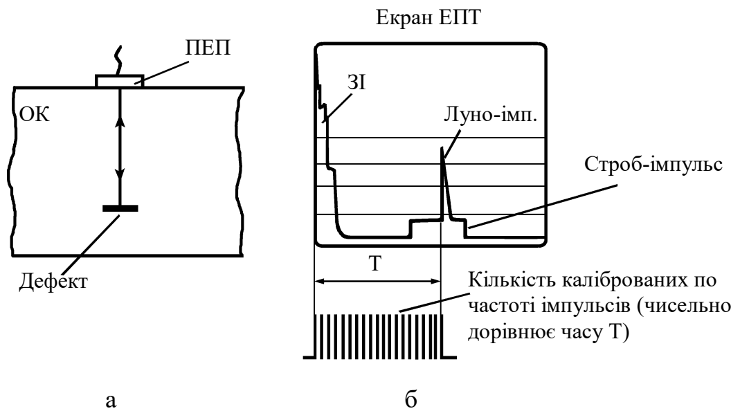
Рис. 4.1. Схема приймання відбитого сигналу для прямого ПЕП
