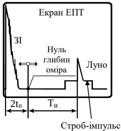
Рис. 4.5. Схема екрана дефектоскопа при настроюванні глибиноміра
