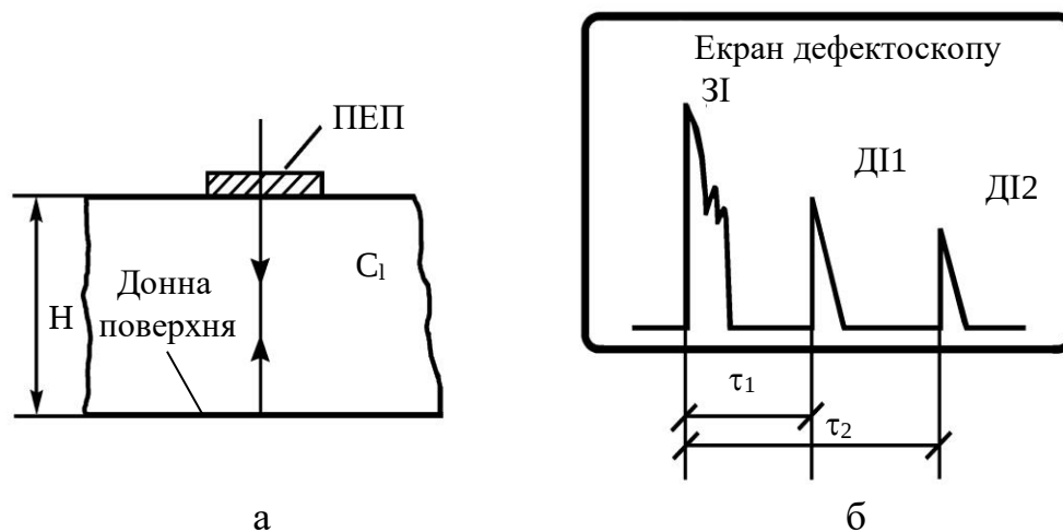
Рис. 1.3. Схема визначення швидкості поздовжньої хвилі за допомогою прямого ПЕП
