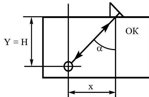
Рис. 1.2. Схема проходження поперечної хвилі в ОК
