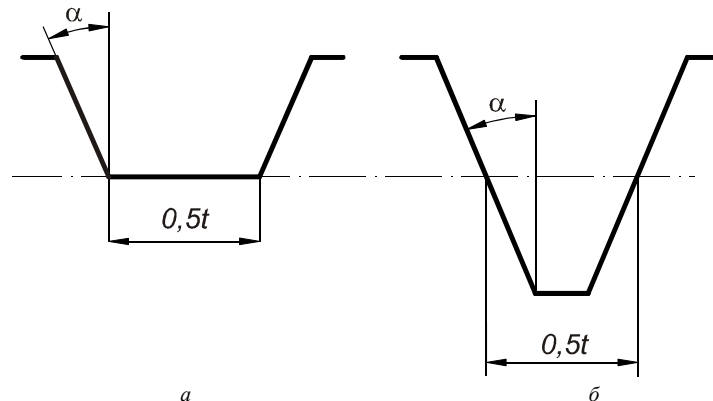
Рис. 5. Прямоугольные гребенки первого (а) и второго (б) прохода
