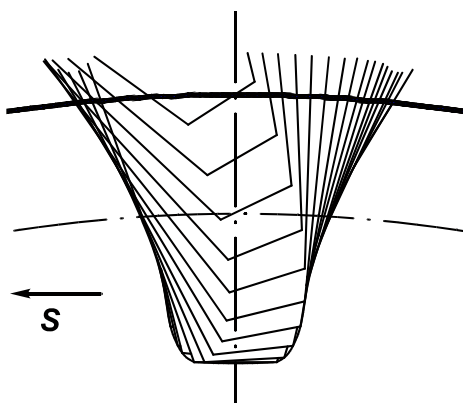
Рис. 3. Схема срезания припуска при однократной обработке
