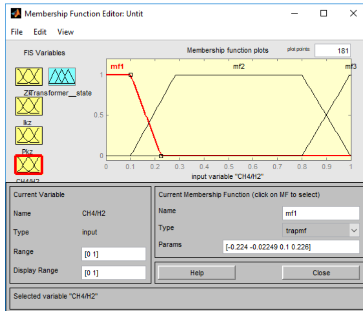
Рисунок 3.9 - Налаштування трапецеїдальної функції CH_4/H_2
