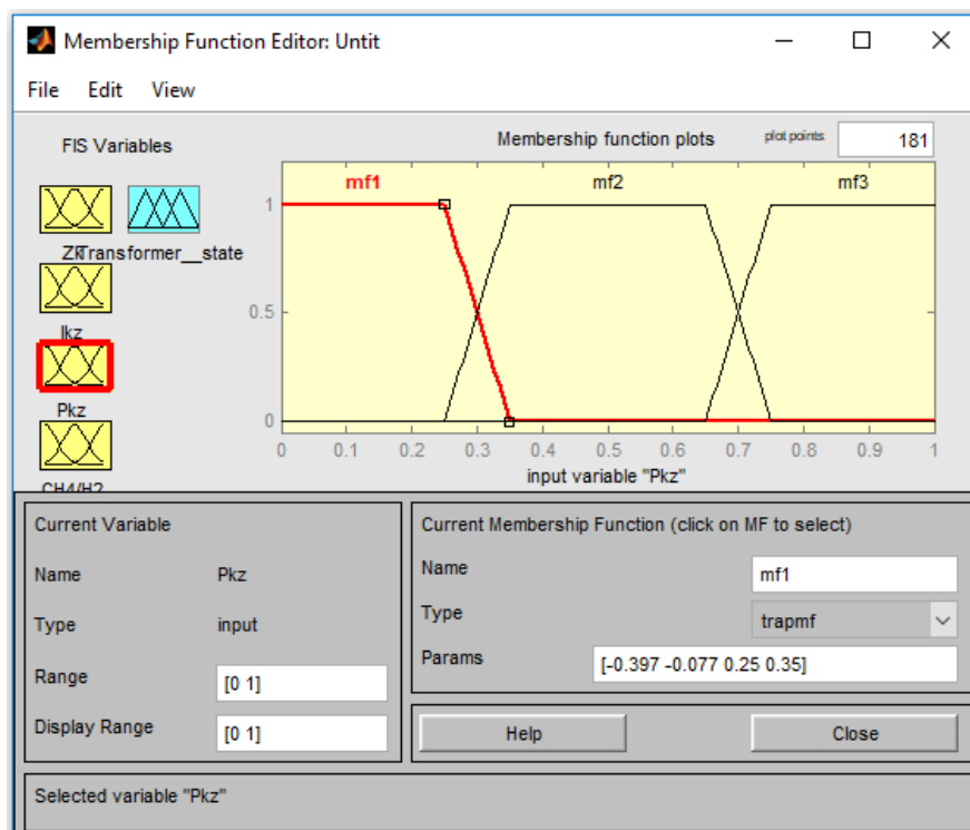
Рисунок 3.6 - Налаштування трапецеїдальної функції P_{к3}
