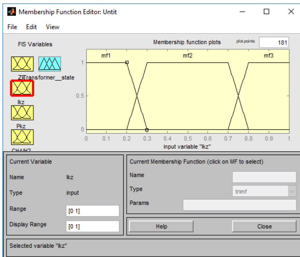
Рисунок 3.8 - Налаштування трапецеїдальної функції I_{K3}
