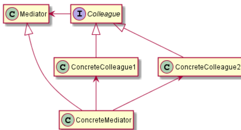
Рис. 2.6. Діаграма класів для шаблону проектування Медіатор
