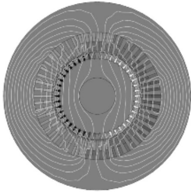
Рис. 1 – Активна зона досліджуваного АД
