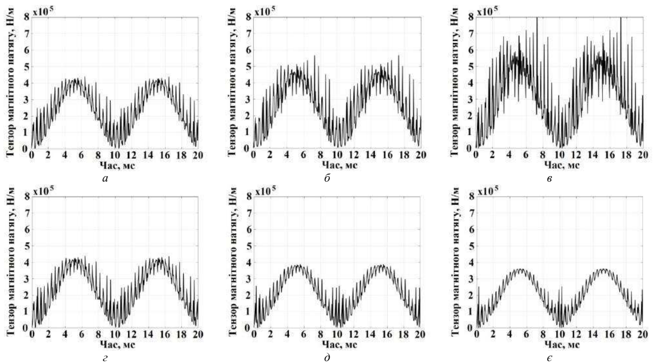
Рис. 2 – Розподіл вібробуджуючих сил в точках з мінімальним (а–в) і з максимальним (з–є) повітряними проміжками при різних величинах k_\phi : а, з) неушкоджений АД, k_\phi = 0 ; б, д) k_\phi = 0,47 ; в, є) k_\phi = 0,91
