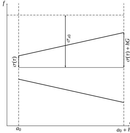
Рис. 2 – Измерение в двух точках: a_0 и a_0 + h
