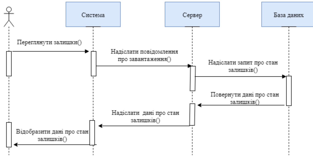
Схема структурна послідовності процесу відображення залишків товарів споживача
