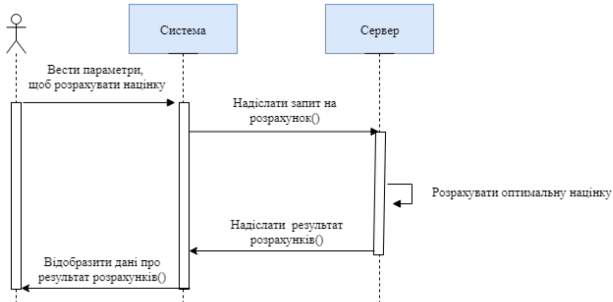
Схема структурна послідовності процесу розрахунку оптимальної націнки
