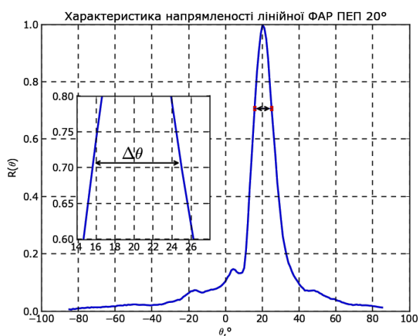
Рис. 9. Експериментальні просторові та часові характеристики УЗ лінійної ФАР при сумісному збудженні п'єзоперетворювачів для кутів \theta=0^\circ та \theta=20^\circ
