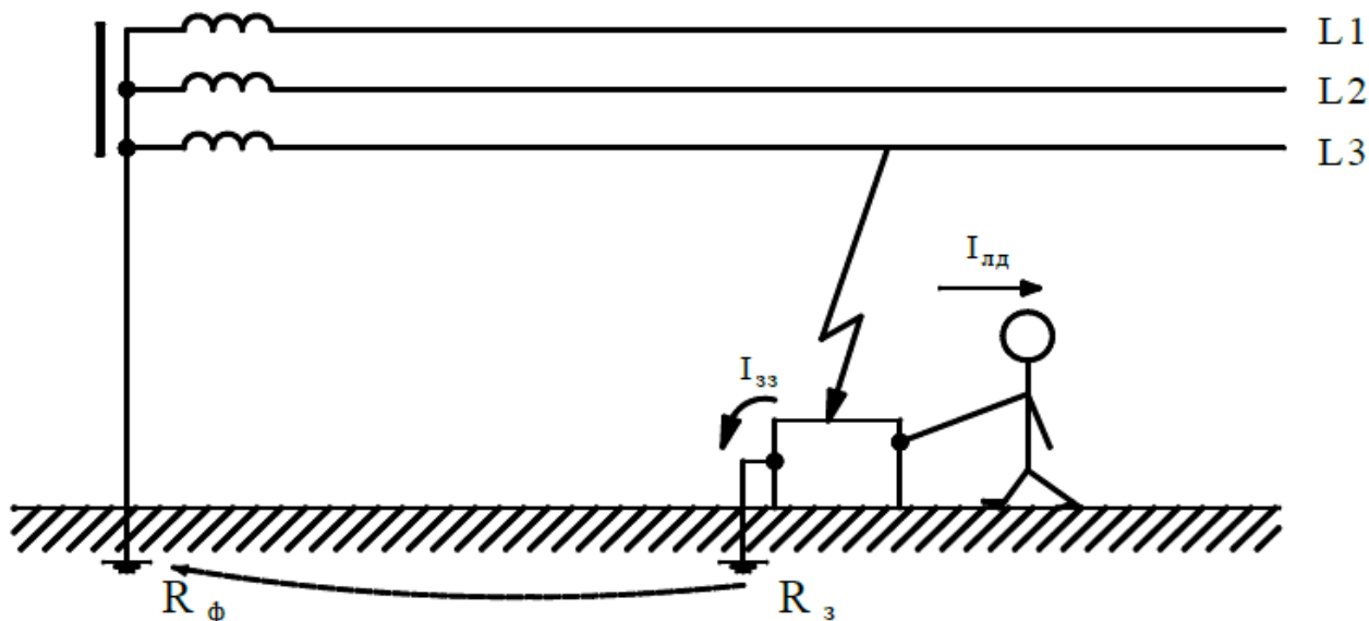
Рис.10.4. Схема захисного заземлення у мережі із заземленою нейтраллю ДЖ (система ТТ)
