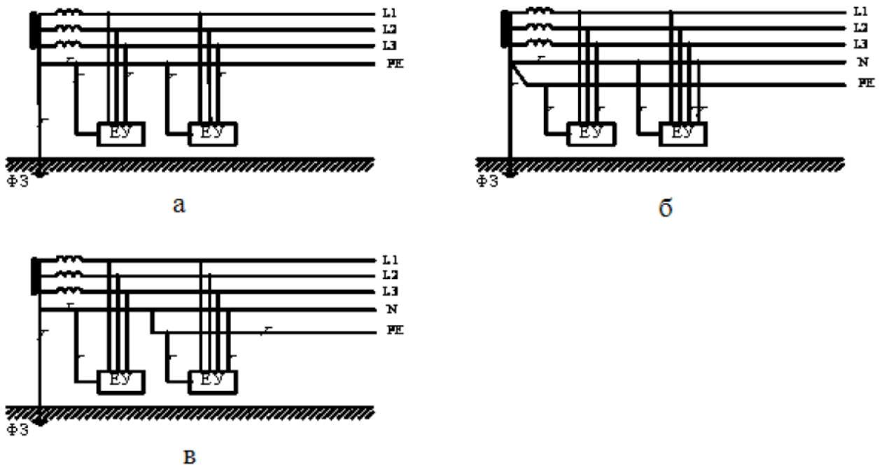
Рис.10.3. Схеми підсистем захисного заземлення системи ТN в ЕУ напругою до 1 кВ: а – підсистеми ТN-С; б – підсистеми ТN-S; в – підсистеми ТN-C-S
