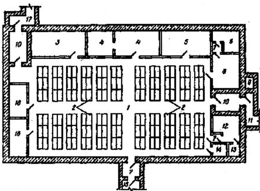
Рис. 13.1. План сховища:
