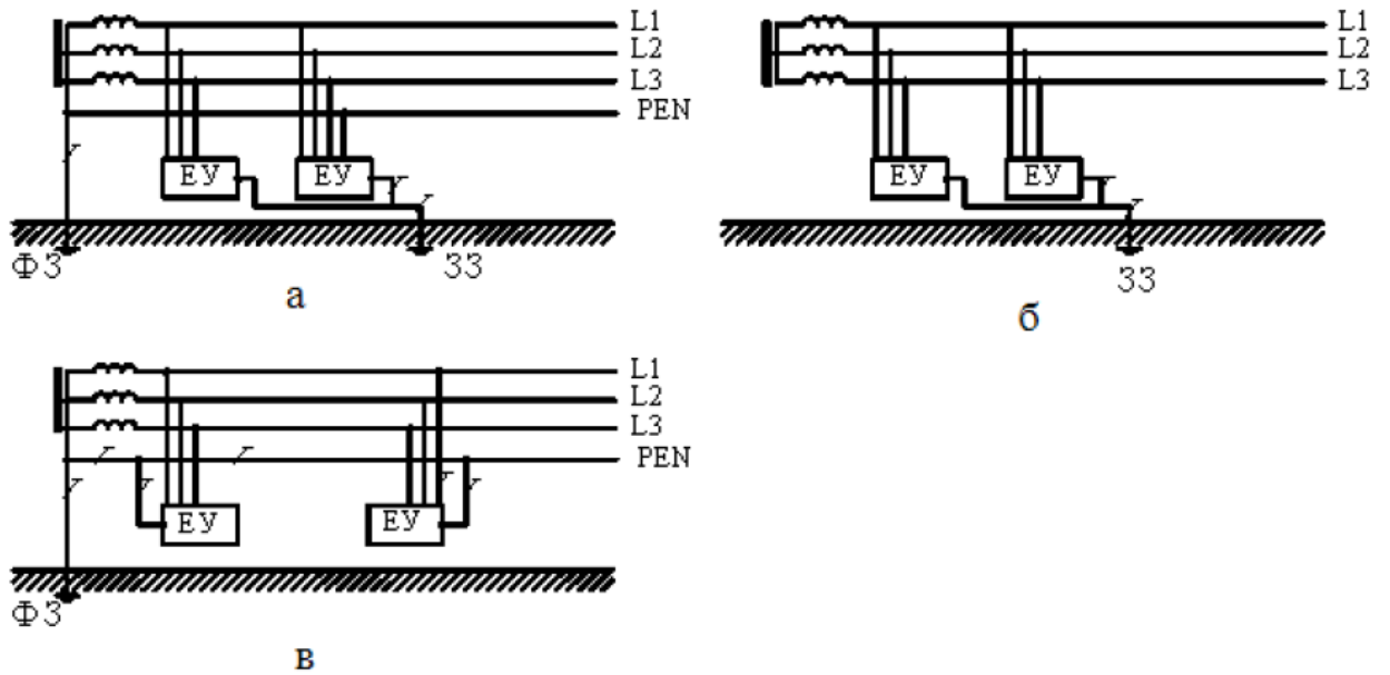
Рис.10.2. Схеми систем заземлення в ЕУ напругою до 1 кВ: а – типу ТТ; б – типу ІТ; в – типу ТN; ФЗ – функціональне зазелення; ЗЗ – захисне заземлення
