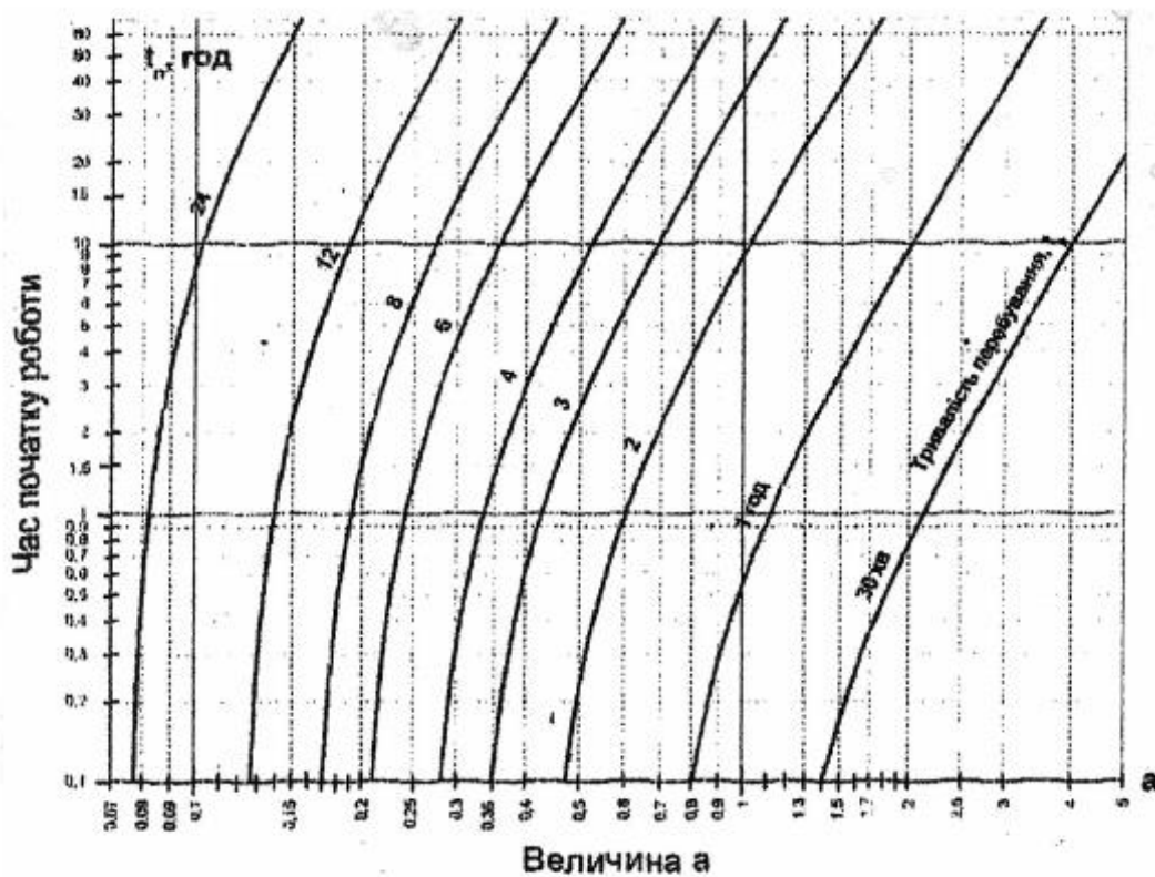
Рис 14.2. Графік визначення тривалості перебування в зоні радіоактивного зараження при аварії на АЕС з реактором РБМК-1000
