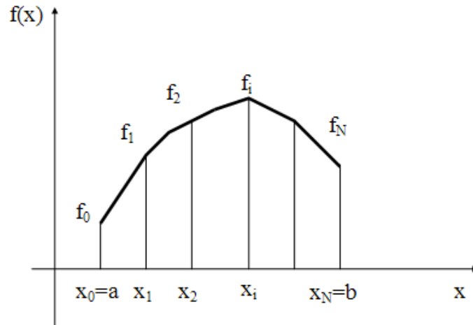
Рис. 2. Поліноміальний сплайн
