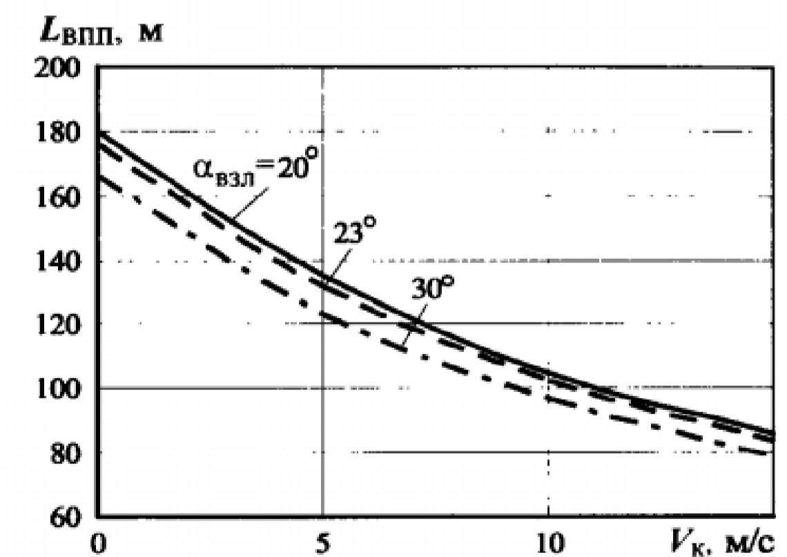
Необхідна довжина взлітно-посадкової смуги
