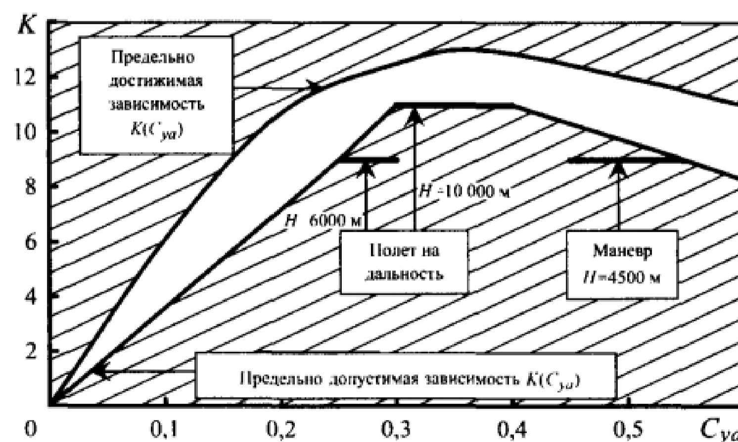
Вимоги до аеродинамічної якості для тренажерного літака
