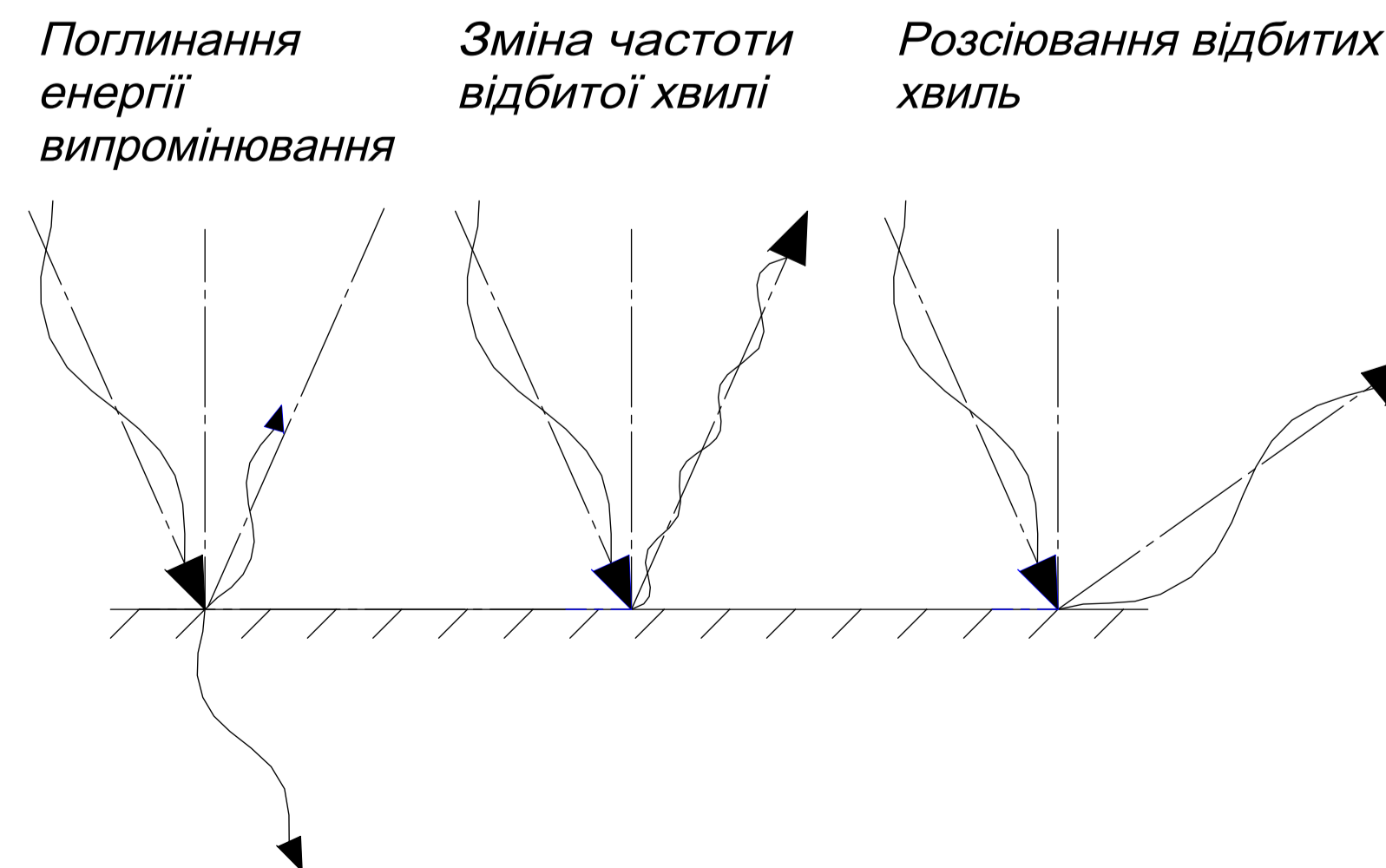
Нанесення радіо поглинаючих поверхонь (принцип їх дії)
