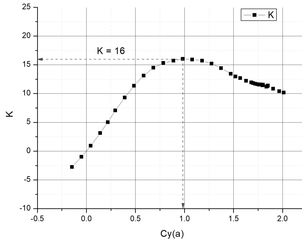
Графік K \backslash C_y для другого варіанту
