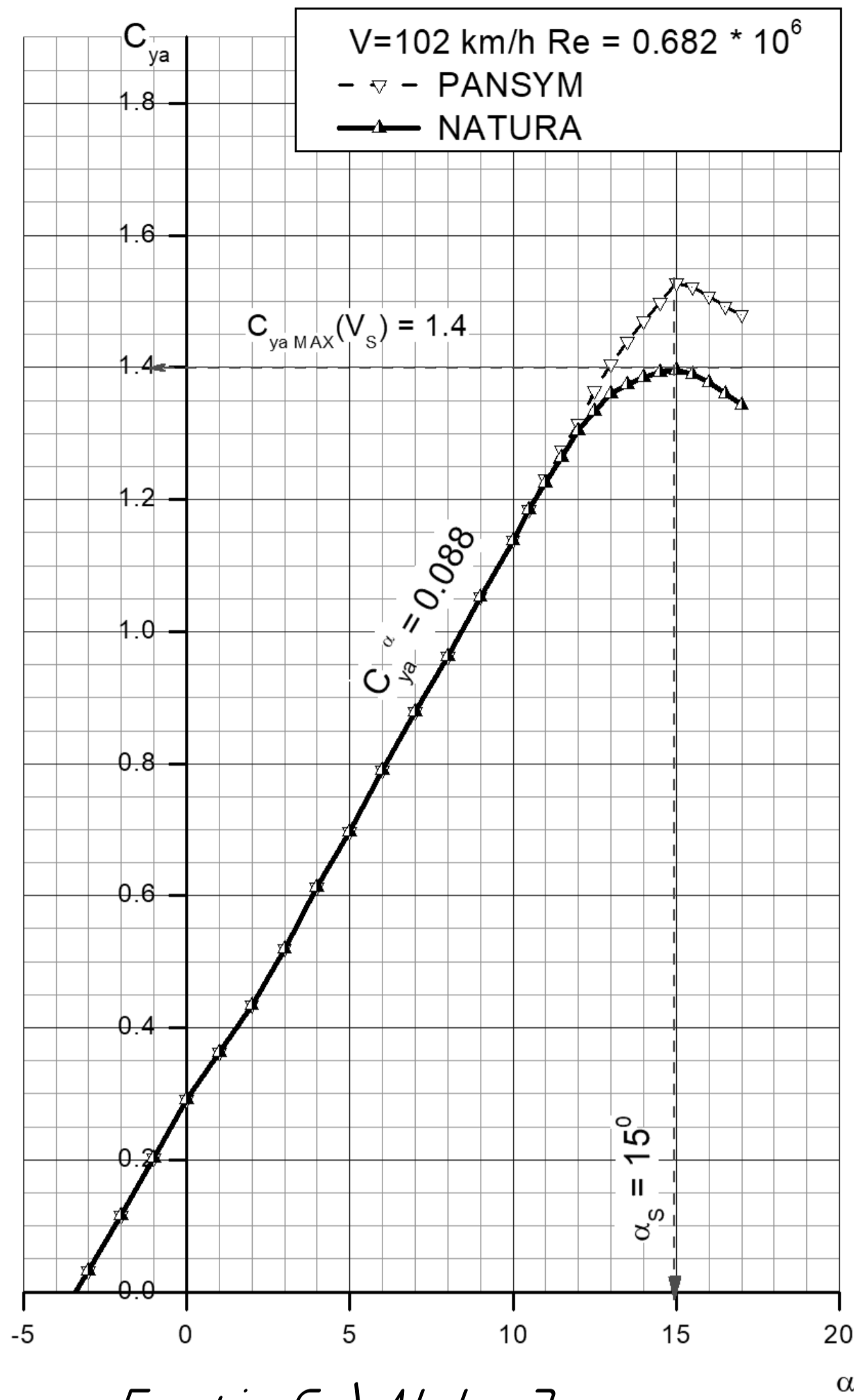
Графік C_y \backslash \alpha для крила та фюзеляжу
