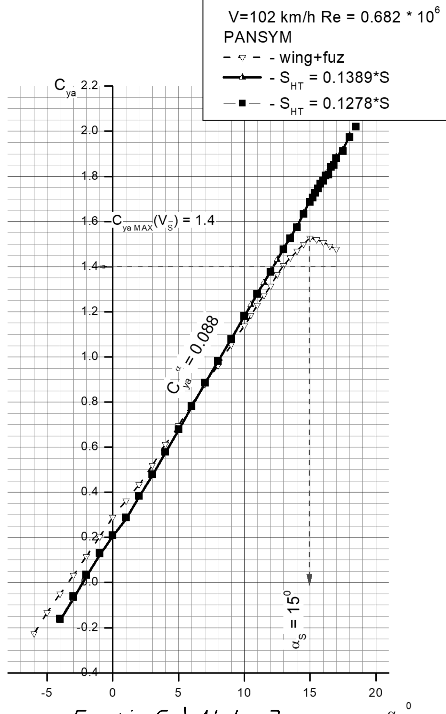
Графік C_y \backslash \alpha для різних видів компонентування
