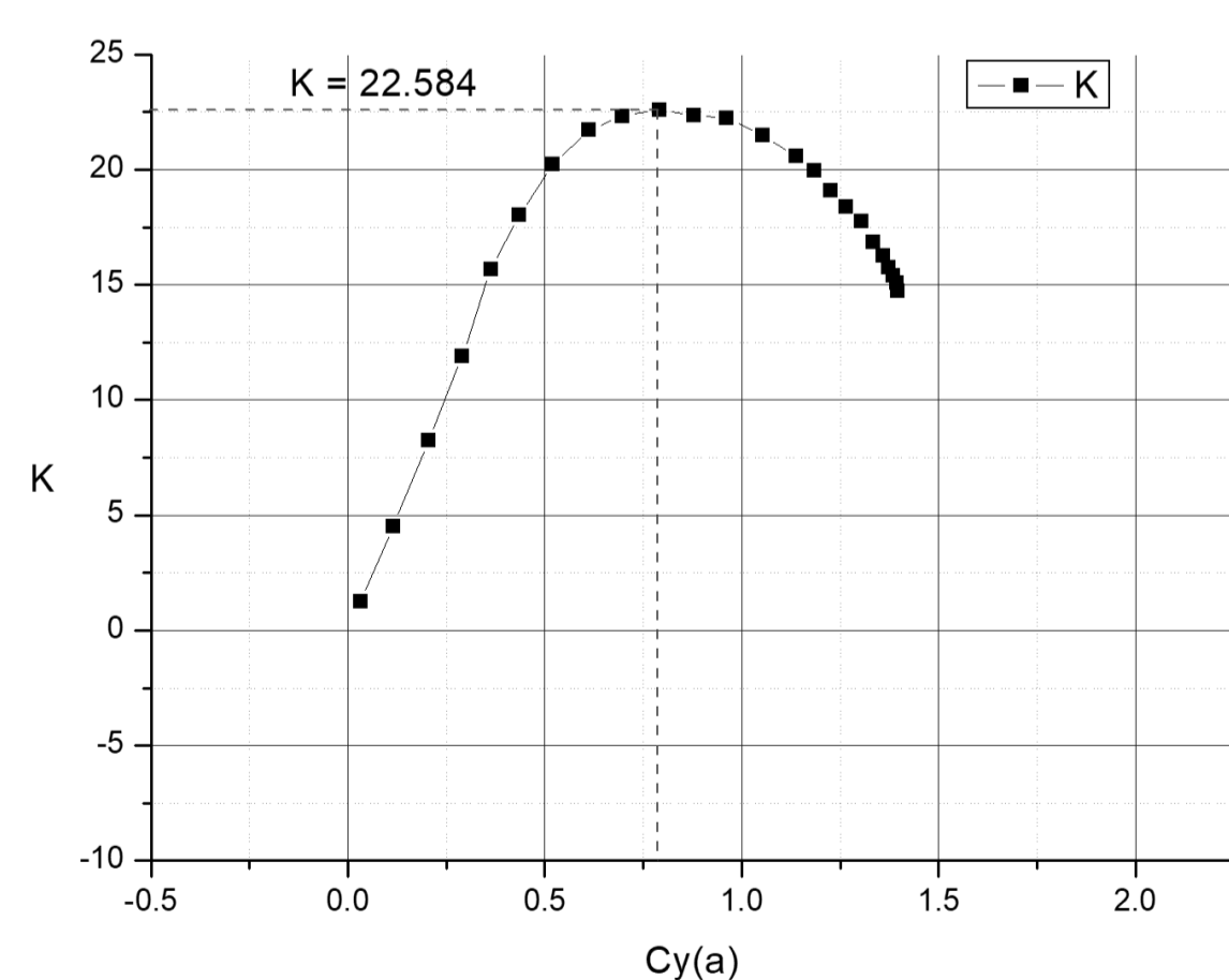
Графік K \backslash C_y для крила та фюзеляжу
