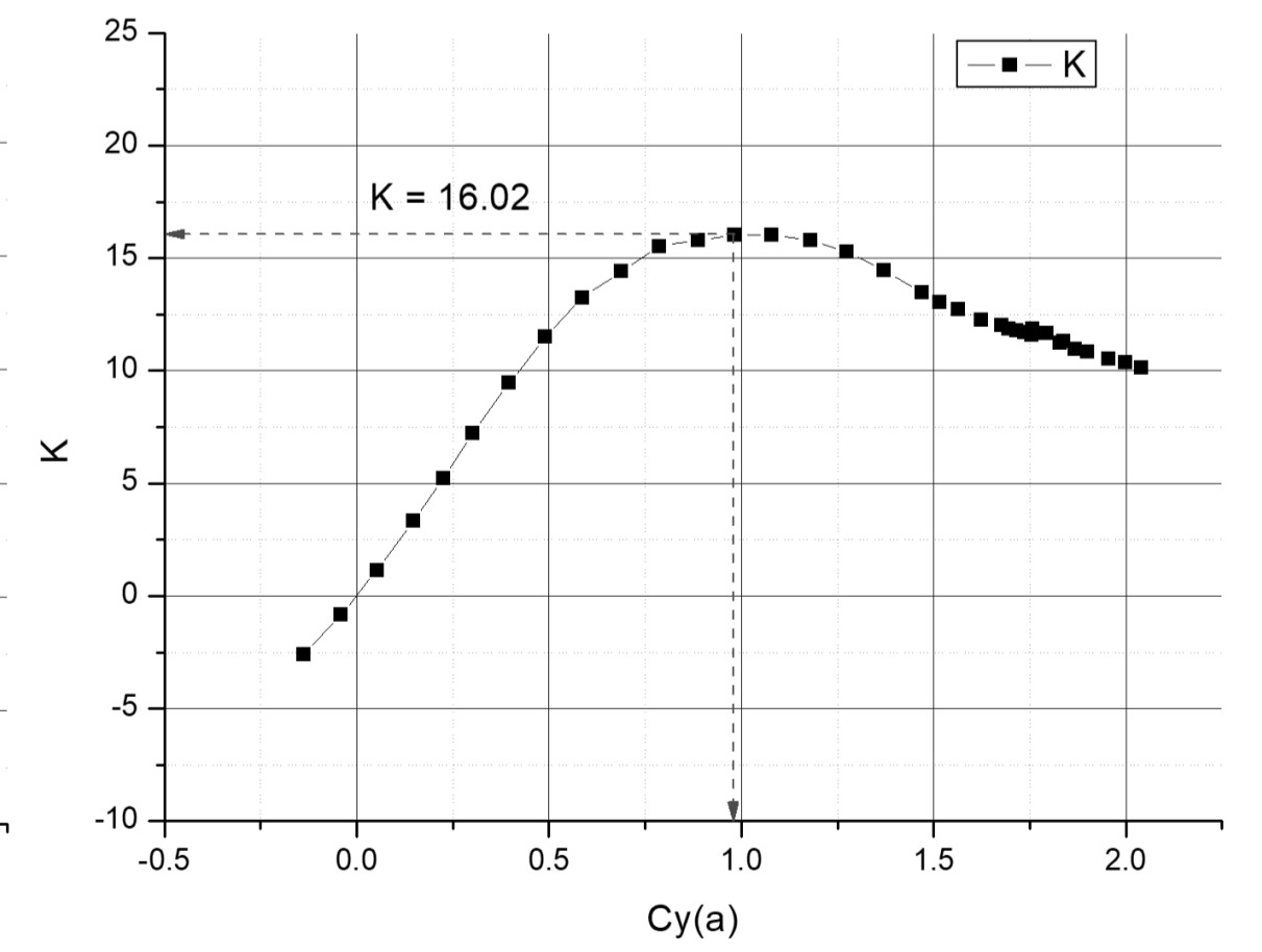
Графік K \backslash C_y для третього варіанту
