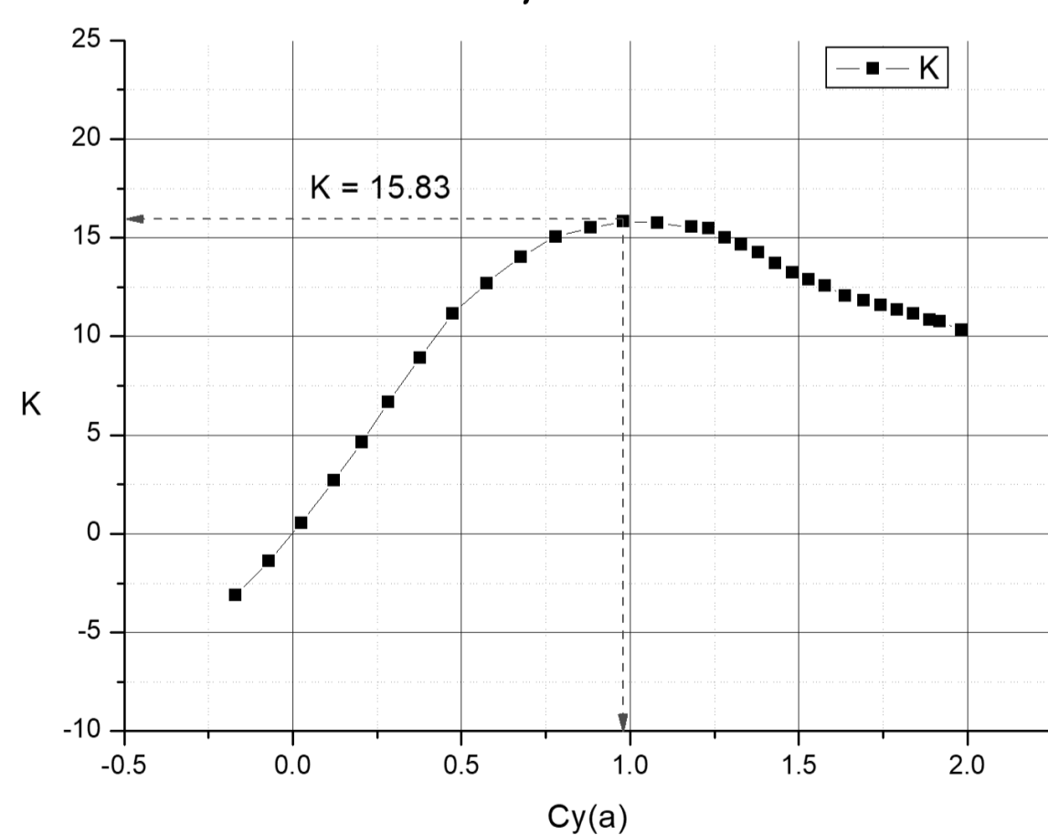
Графік K \backslash C_y для повної компоновки
