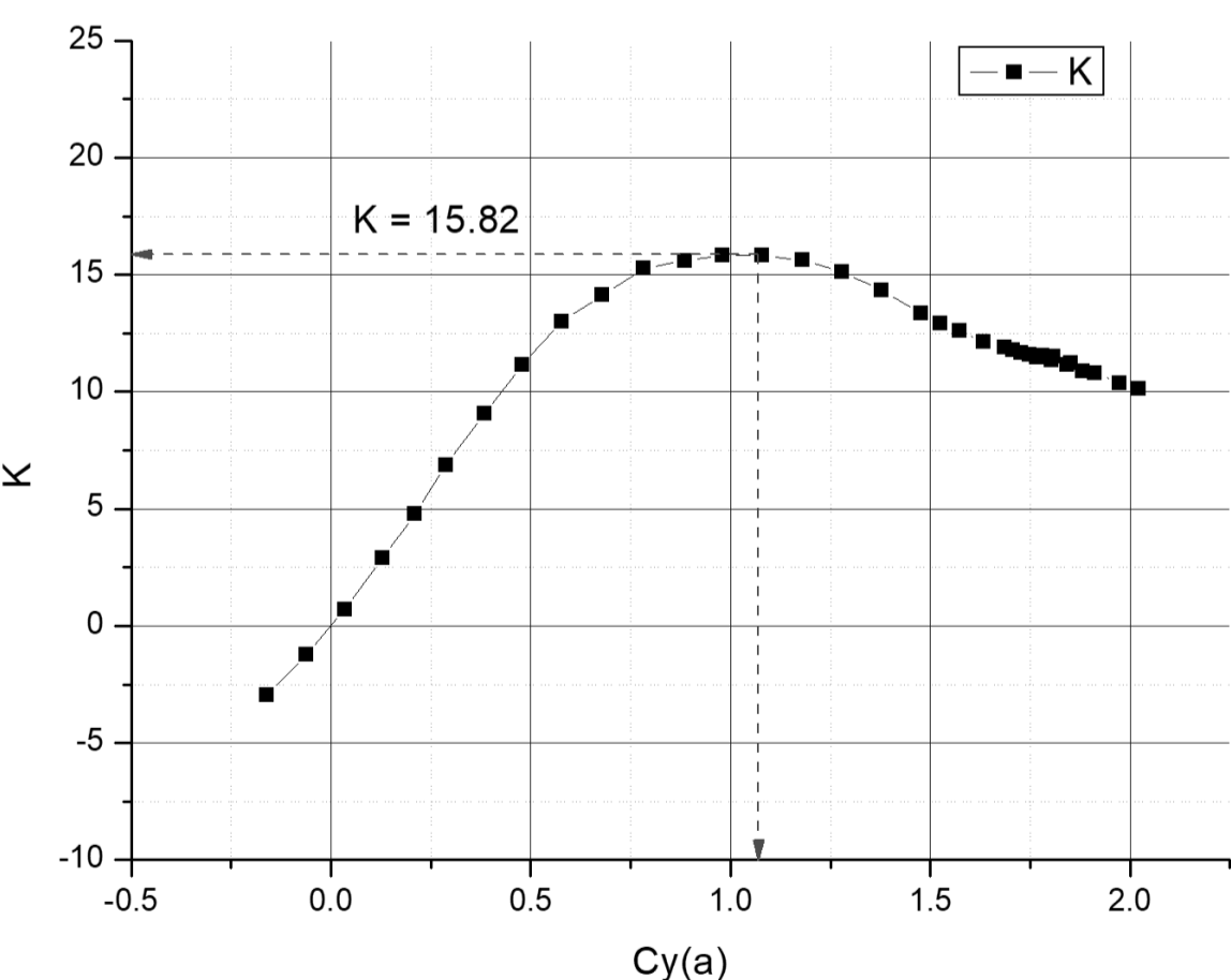
Графік K \backslash C_y для першого варіанту
